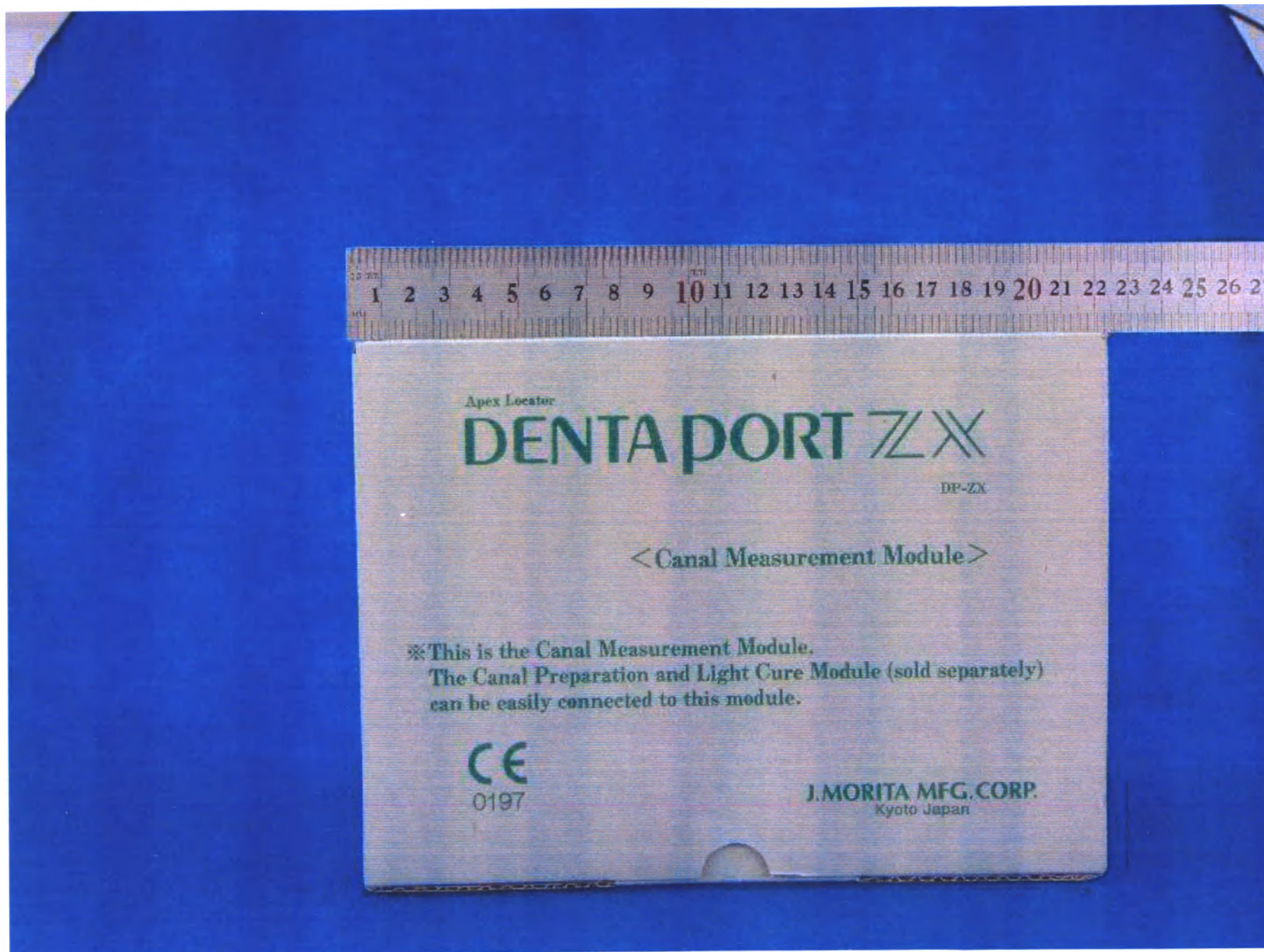
7) Фотография макета упаковки и маркировки медицинского изделия (вид сверху)
