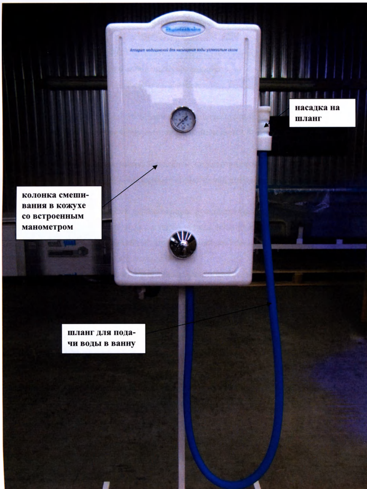
Фотография опытного образца АНУ: общий вид.
