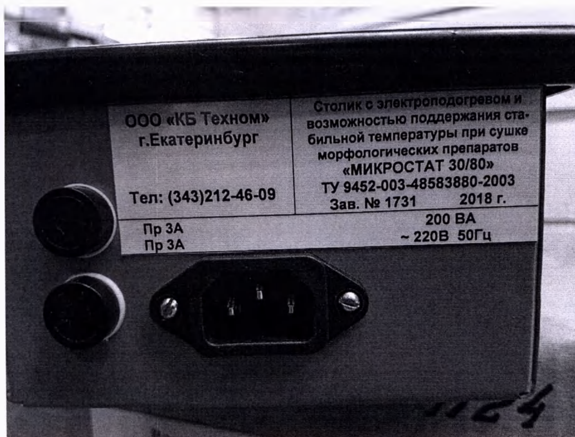
Рис. 2 Столик с электроподогревом и возможностью поддержания стабильной температуры при сушке морфологических препаратов «МИКРОСТАТ-30/80» по ТУ 9452-003-48583880-2003. Маркировка
