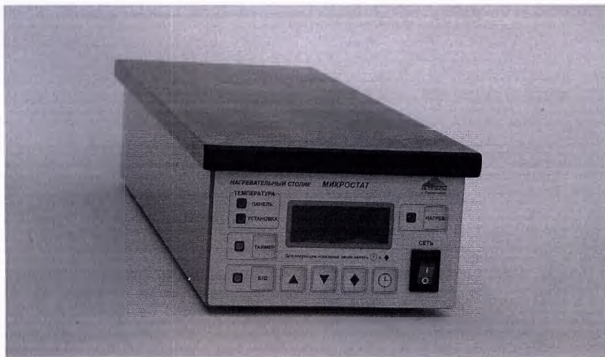
Рис. 1 Столик с электроподогревом и возможностью поддержания стабильной температуры при сушке морфологических препаратов «МИКРОСТАТ-30/80». Внешний вид
