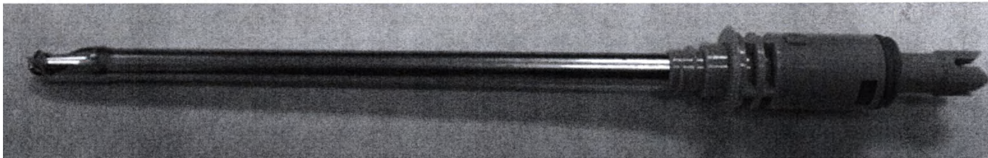
Бур круглый агрессивный 6-крыльчатый 5.5 мм (5 шт. в упаковке)
