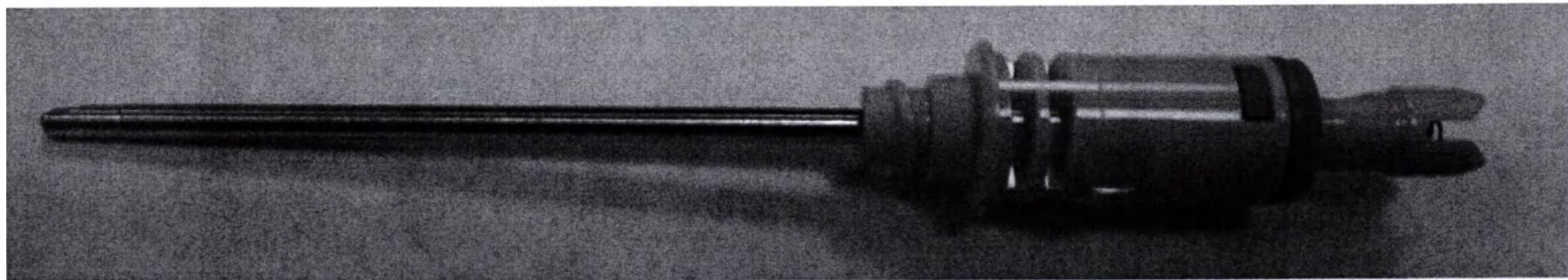
Фреза резекционная полнорadiусная 3.5 мм (5 шт. в упаковке)
