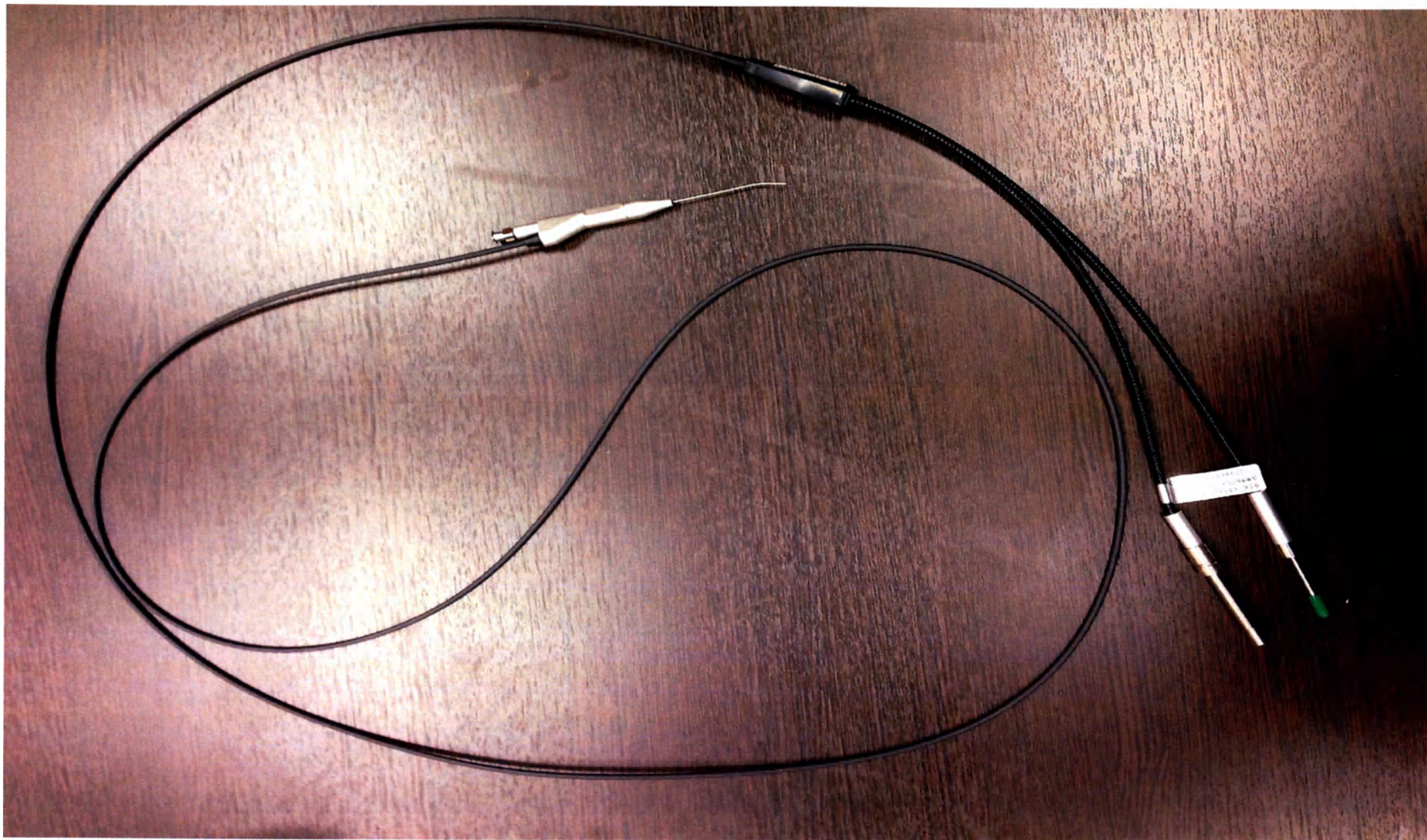
Общий вид эндоскопа слезного канала
