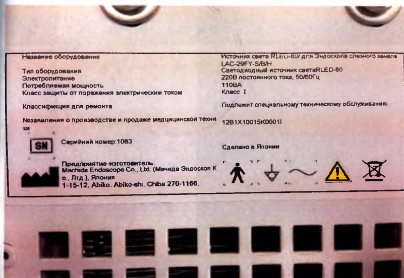
Маркировка источника света
