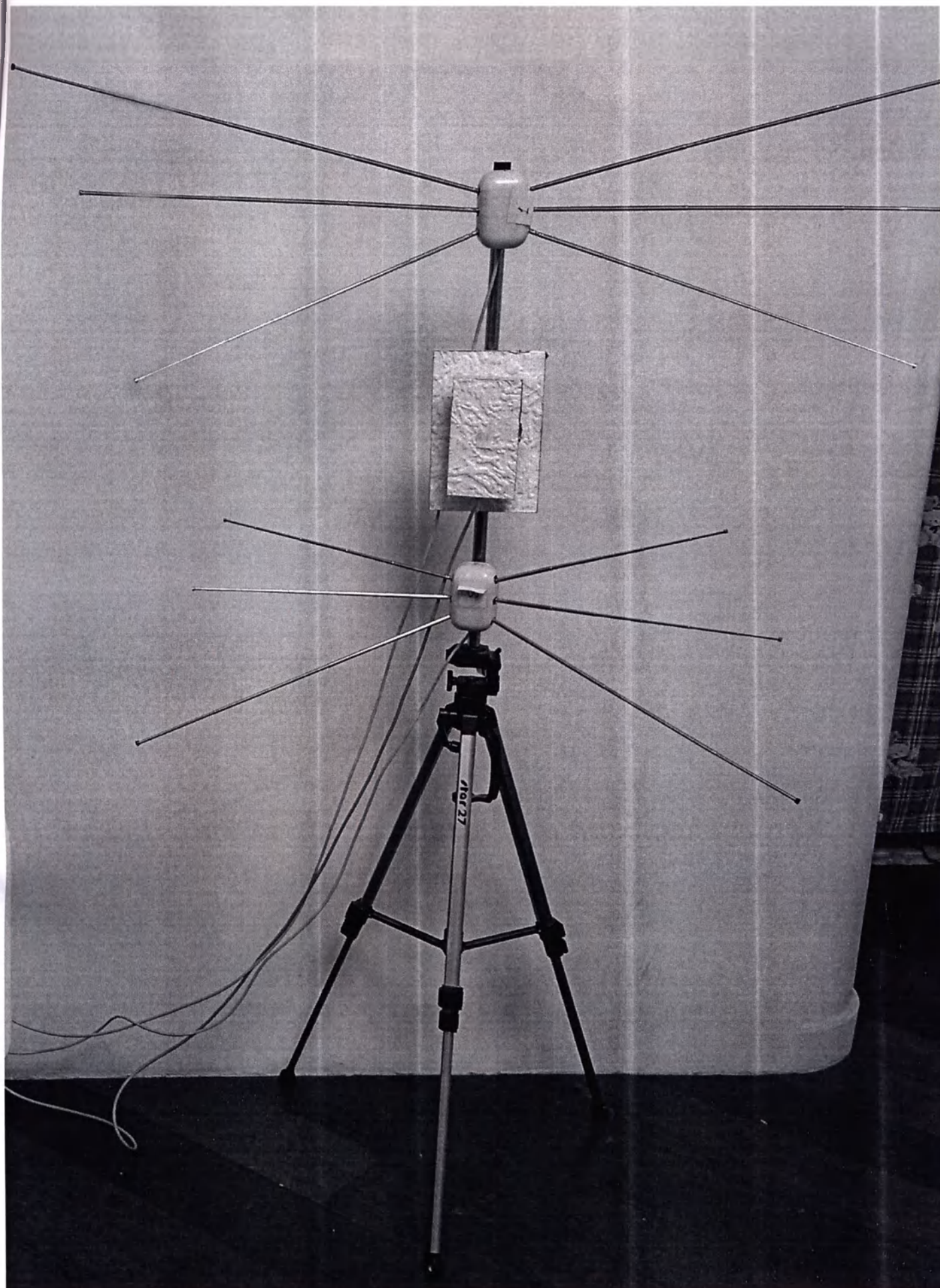
Антенное устройство с волноводами
