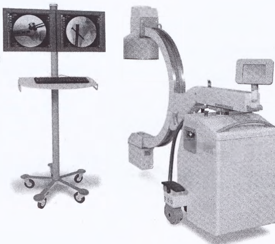
Рис. 3 Внешний вид аппарата. Крепление видеомониторов на стойке
