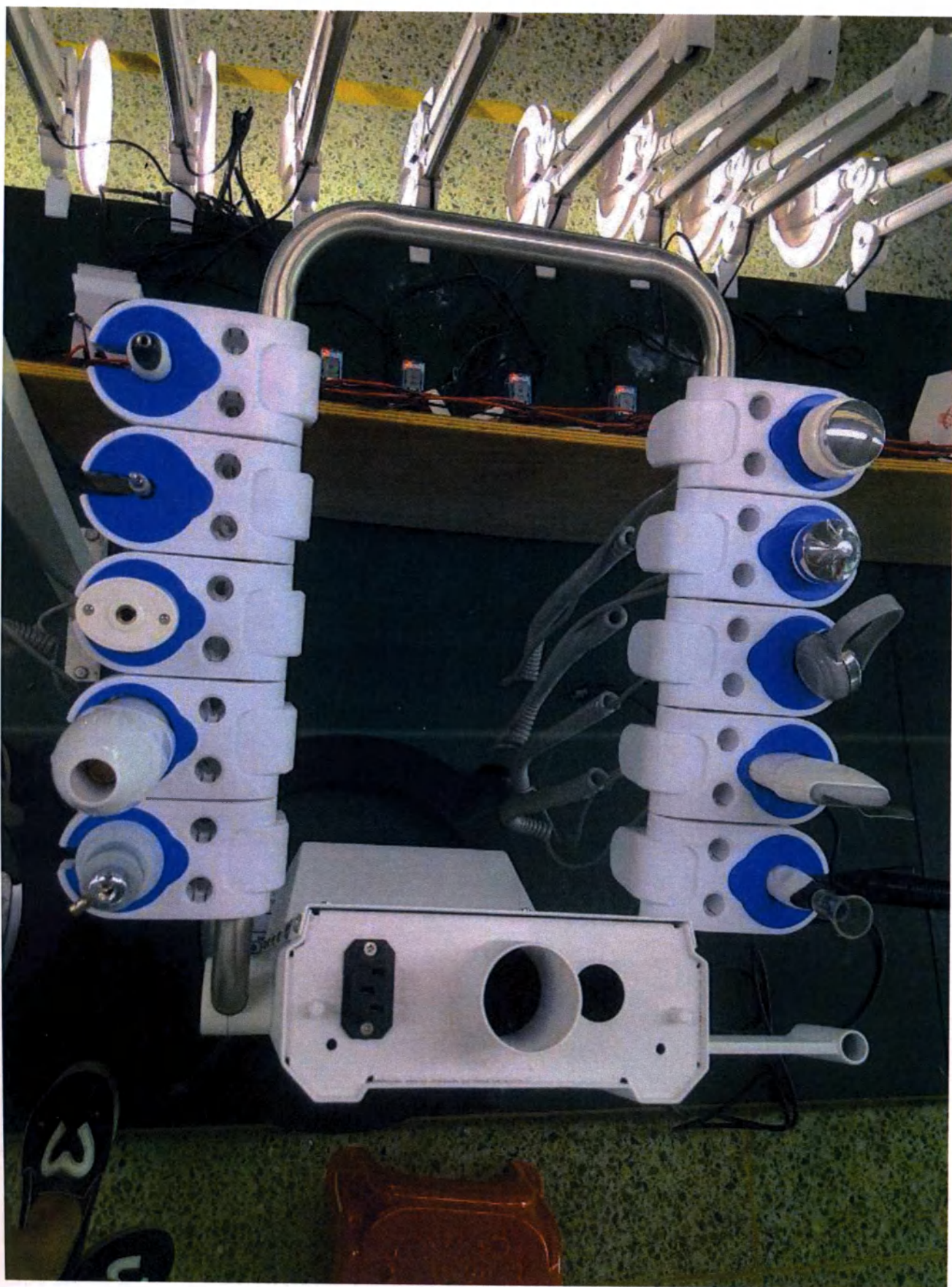
Рисунок 4 - Держатель манипул металлический с пластиковыми пенами
