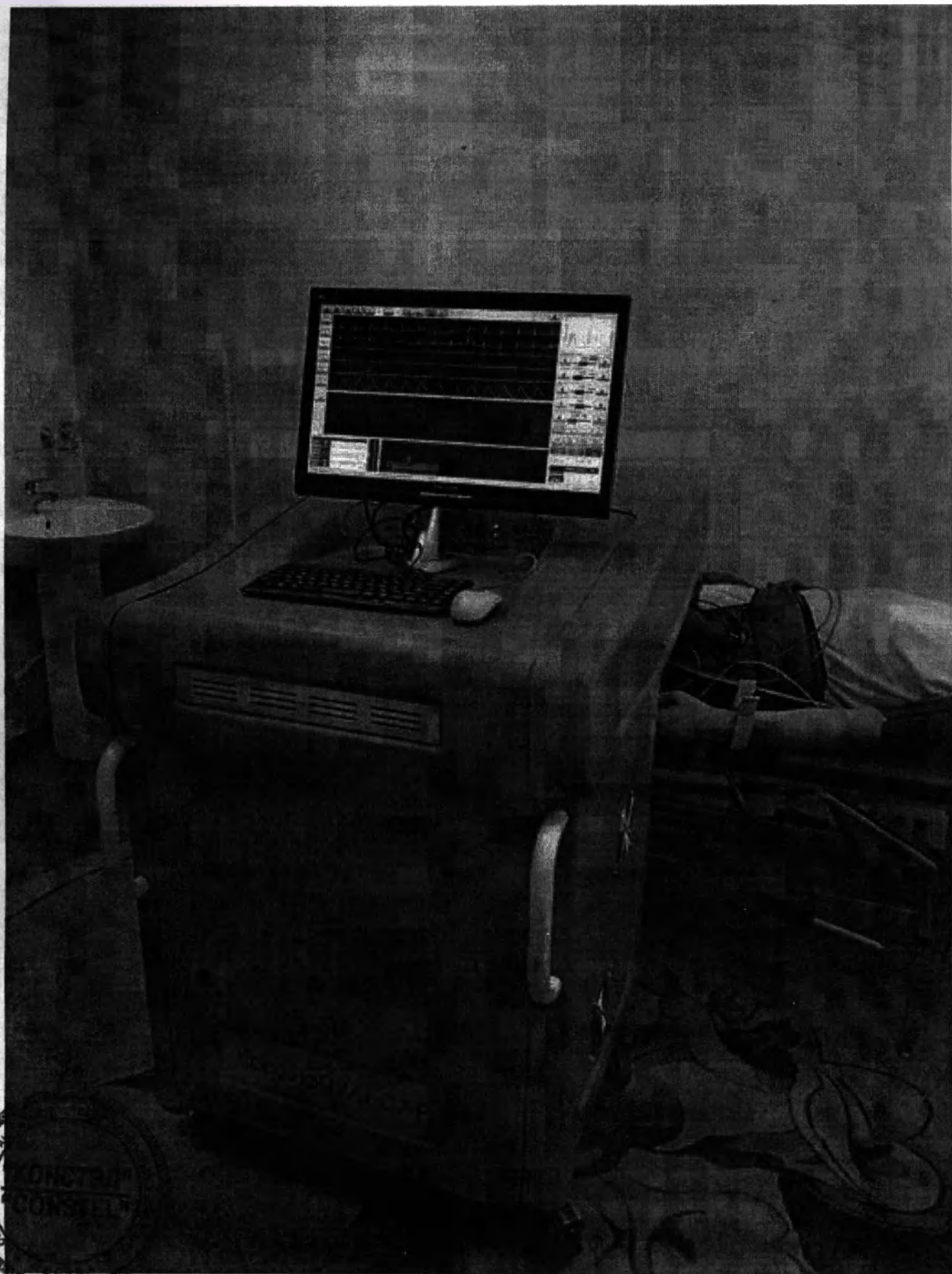
Комплекс программно-аппаратный для вспомогательного кровообращения "КАРДИОПУЛЬСАР" (исполнение М)
