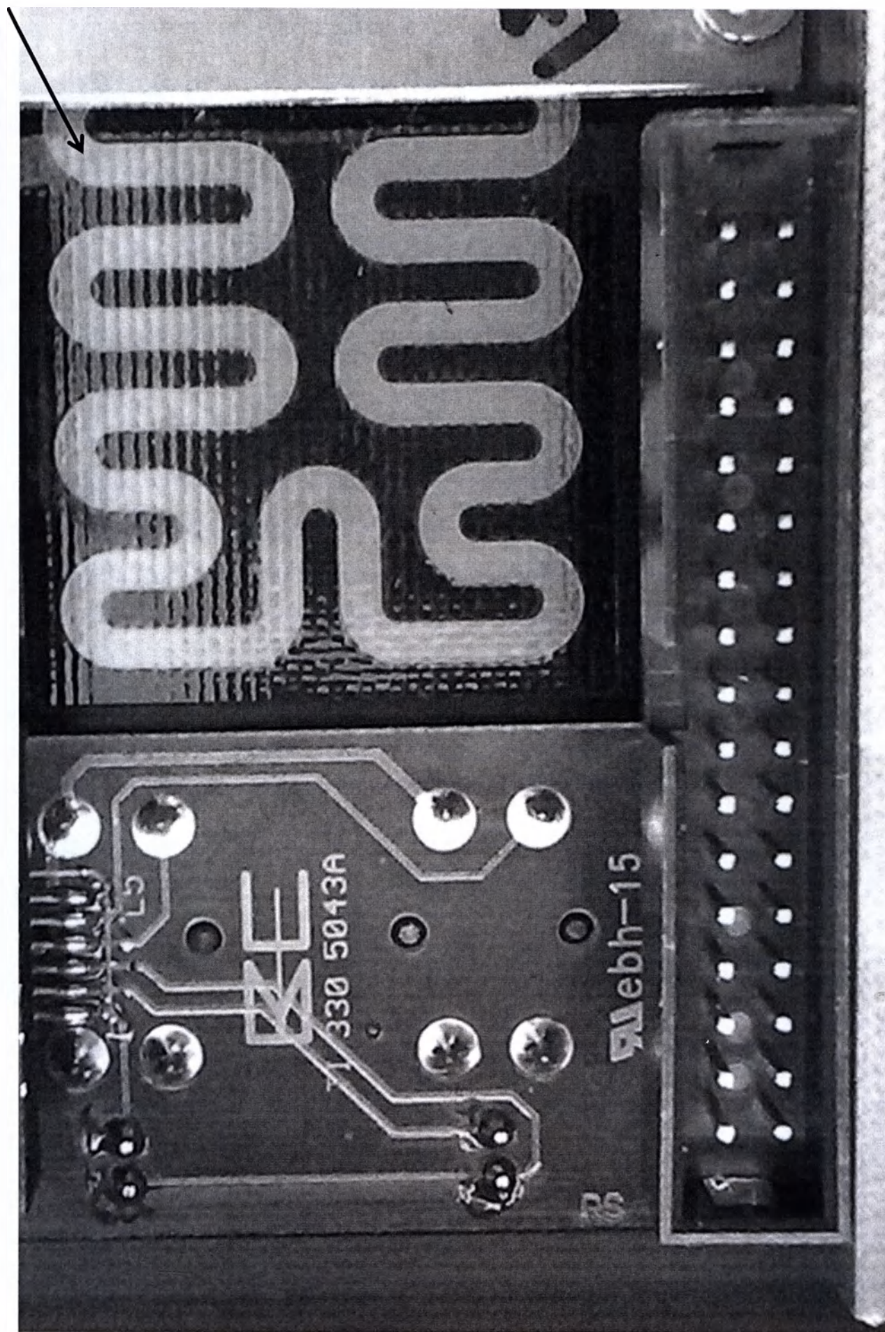
220-008 Резистор нагревателя foil Thrombotimer 4 (показан стрелкой)
