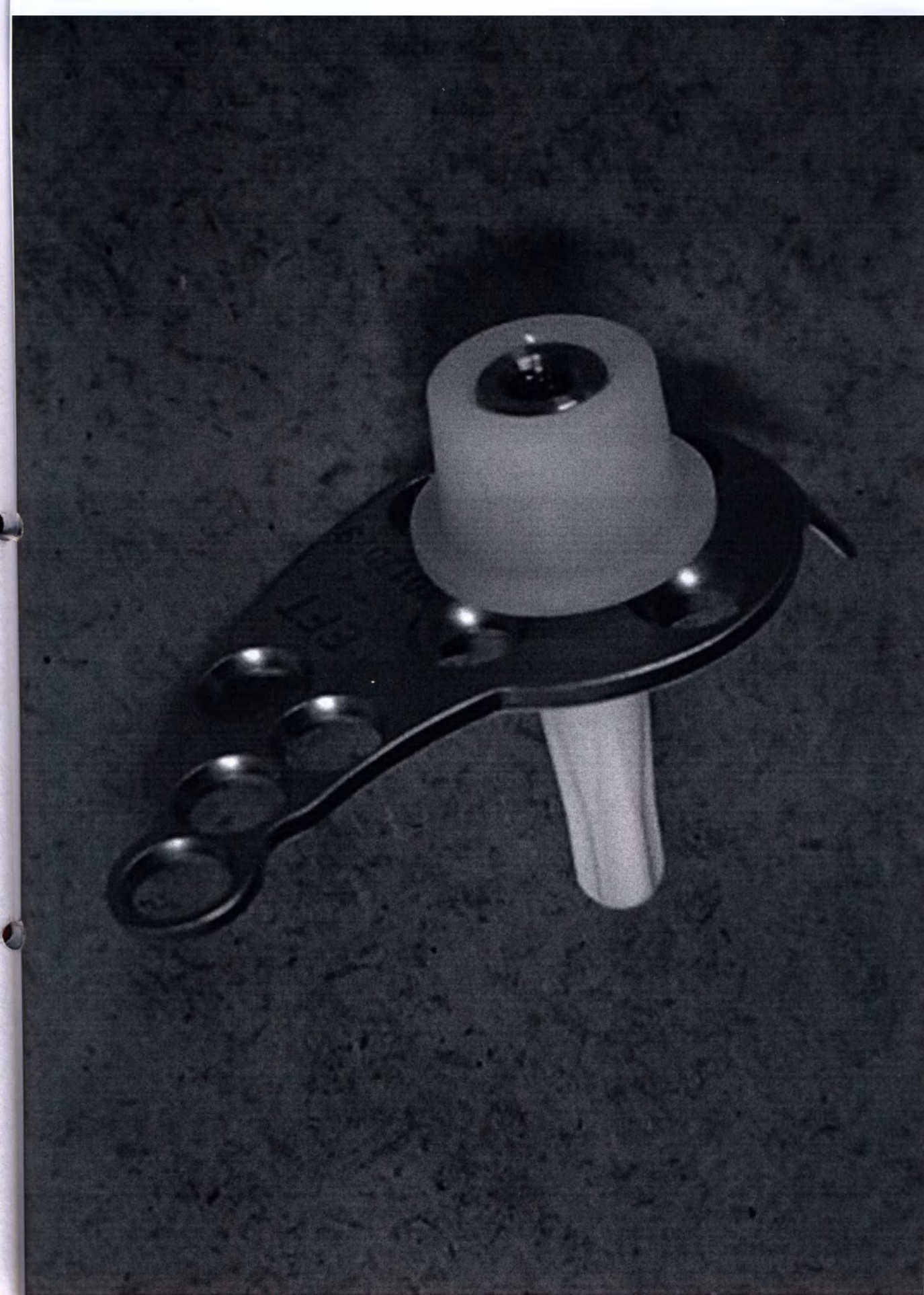
Ревизионное винтовое суставное основание, левое (Revis. HA helical glenoid base Left )
