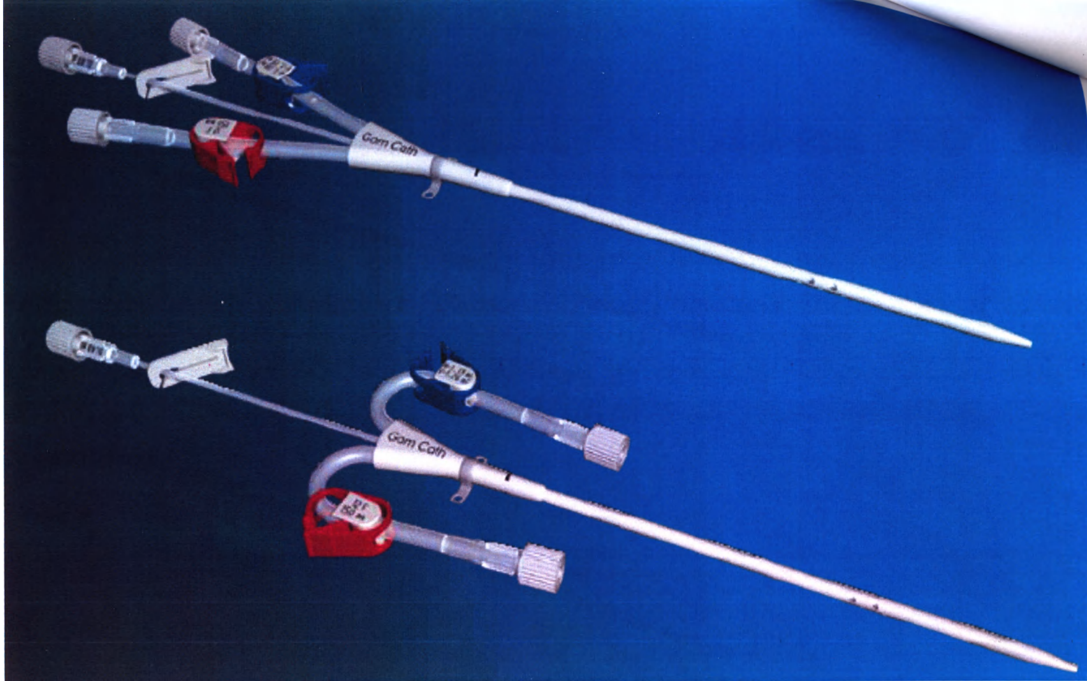
Катетер гемодиализный для сосудистого доступа трехпросветный: GAMCATH, типоразмер GDK (сверху) и GTK (снизу)
