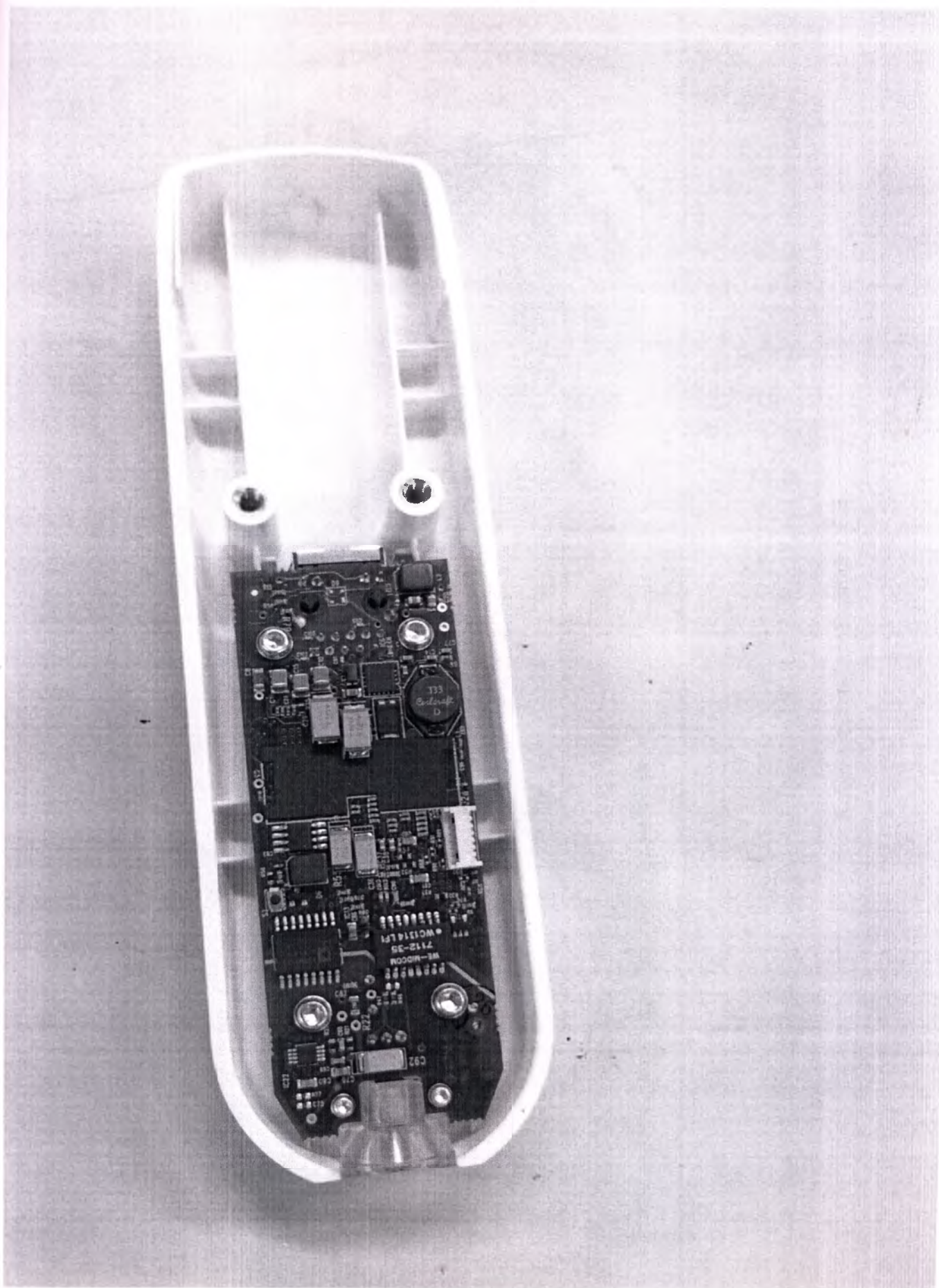
13. Блок управления встраиваемый Planmeca ProSensor
