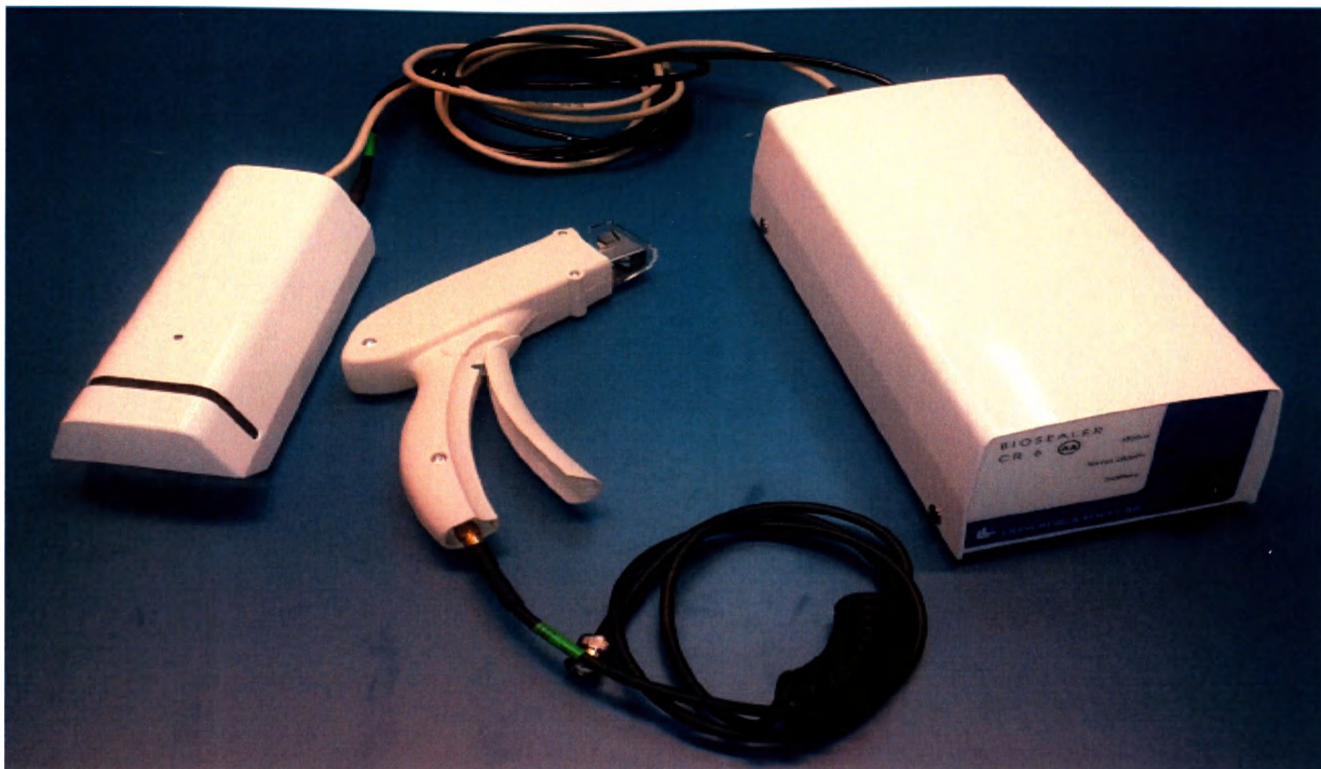
Запаиватель пластиковых магистралей, варианты исполнения: Biosealer CR6 и CR6-AA
