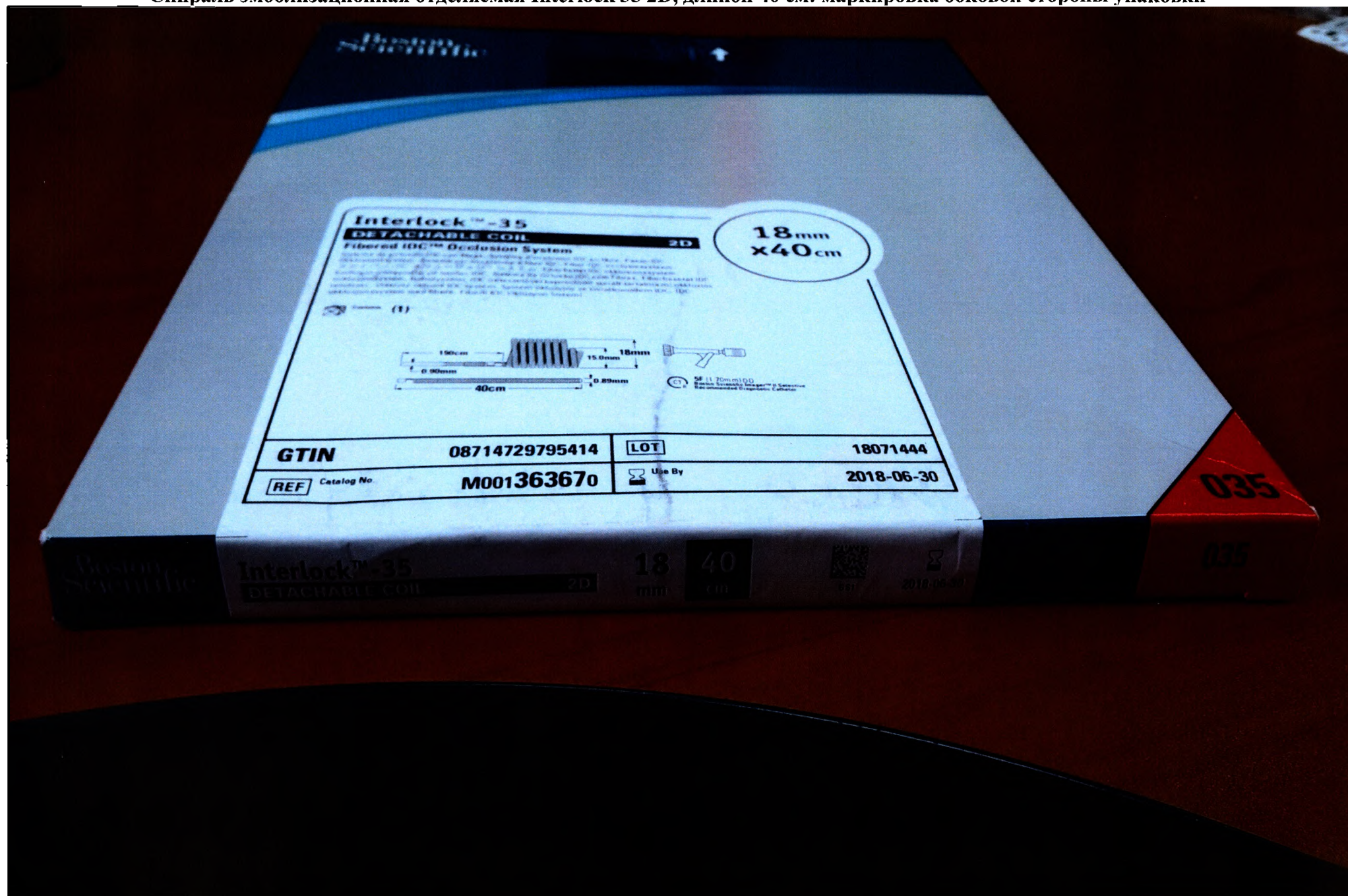
Спираль эмболизационная отделяемая Interlock 35 2D, длиной 40 см: маркировка боковой стороны упаковки
