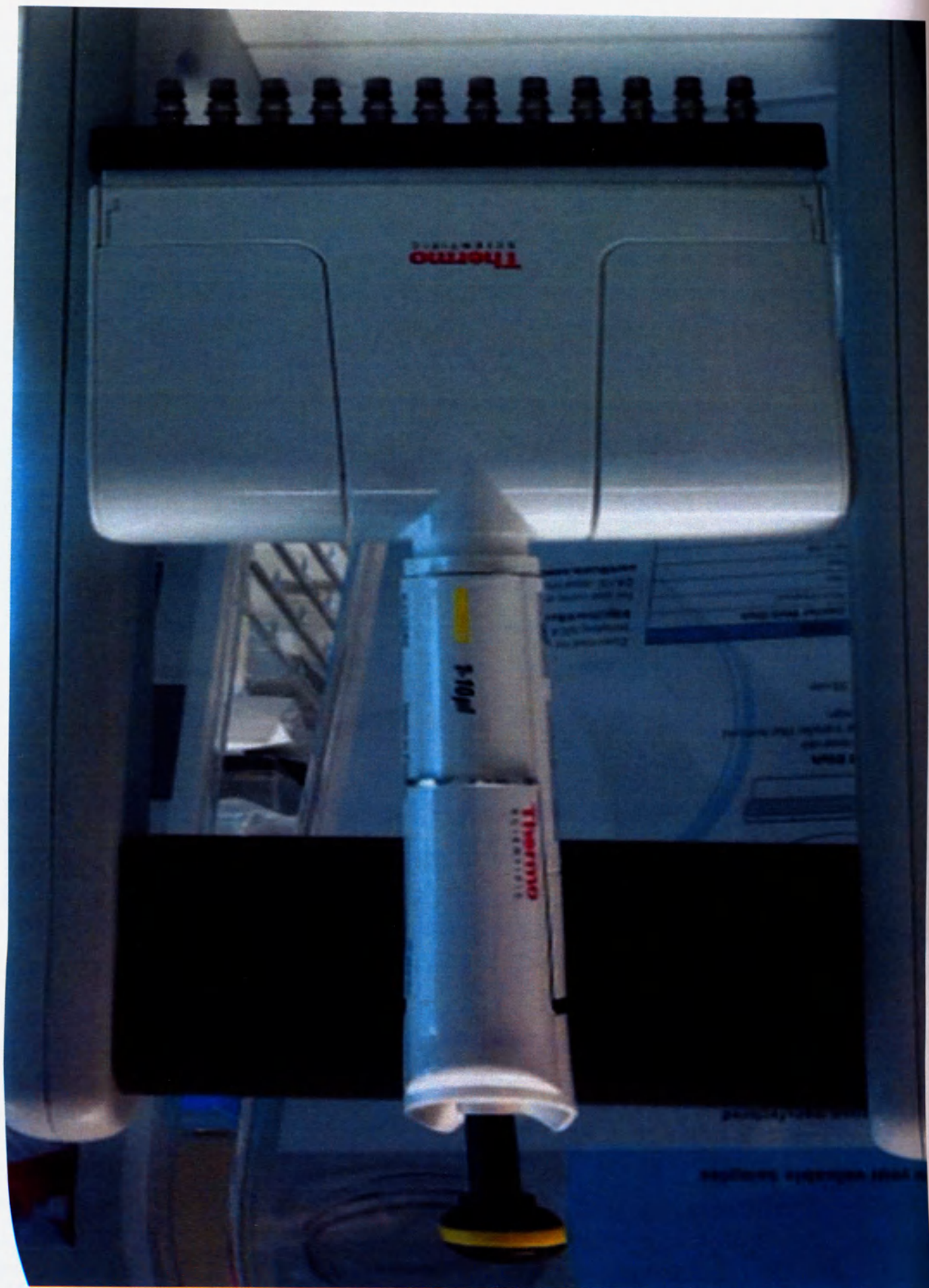
Дозаторы пипеточные F1-ClipTip 12-канальные переменного объема 1-10 мкл
