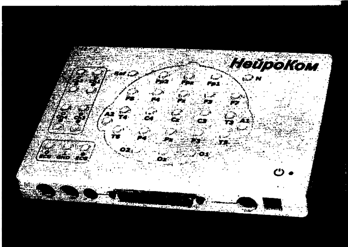
Усилитель биопотенциалов с интерфейсным блоком (УБ)
