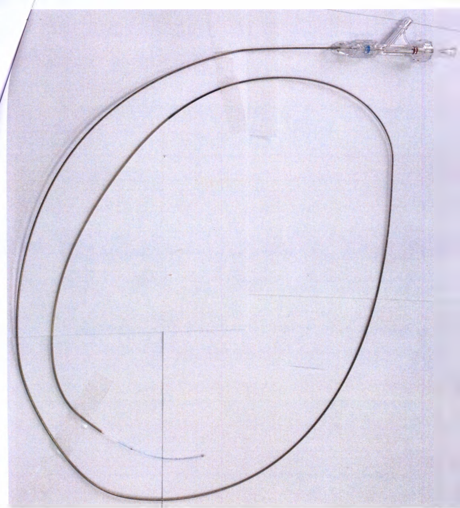
Рис.4. Стент потоко-перенаправляющий для эмболизации аневризм Surpass Flow Diverter система доставки
