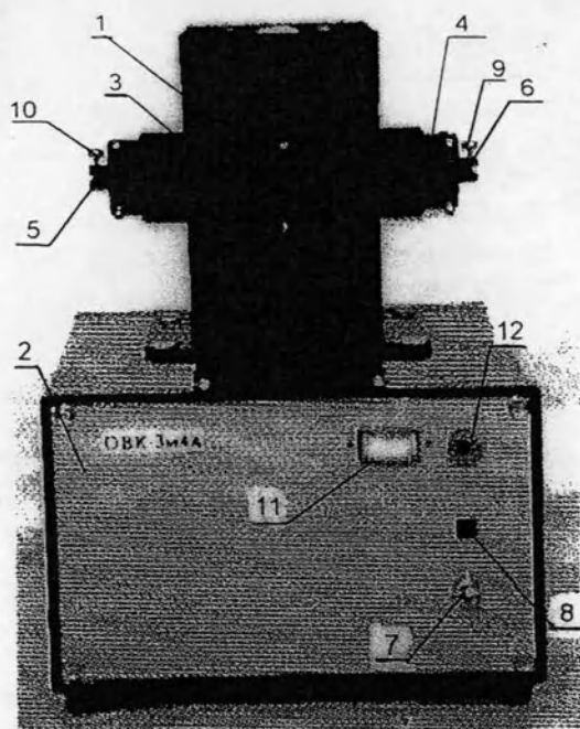
Рис. 1. Облучатель ОВК-3
