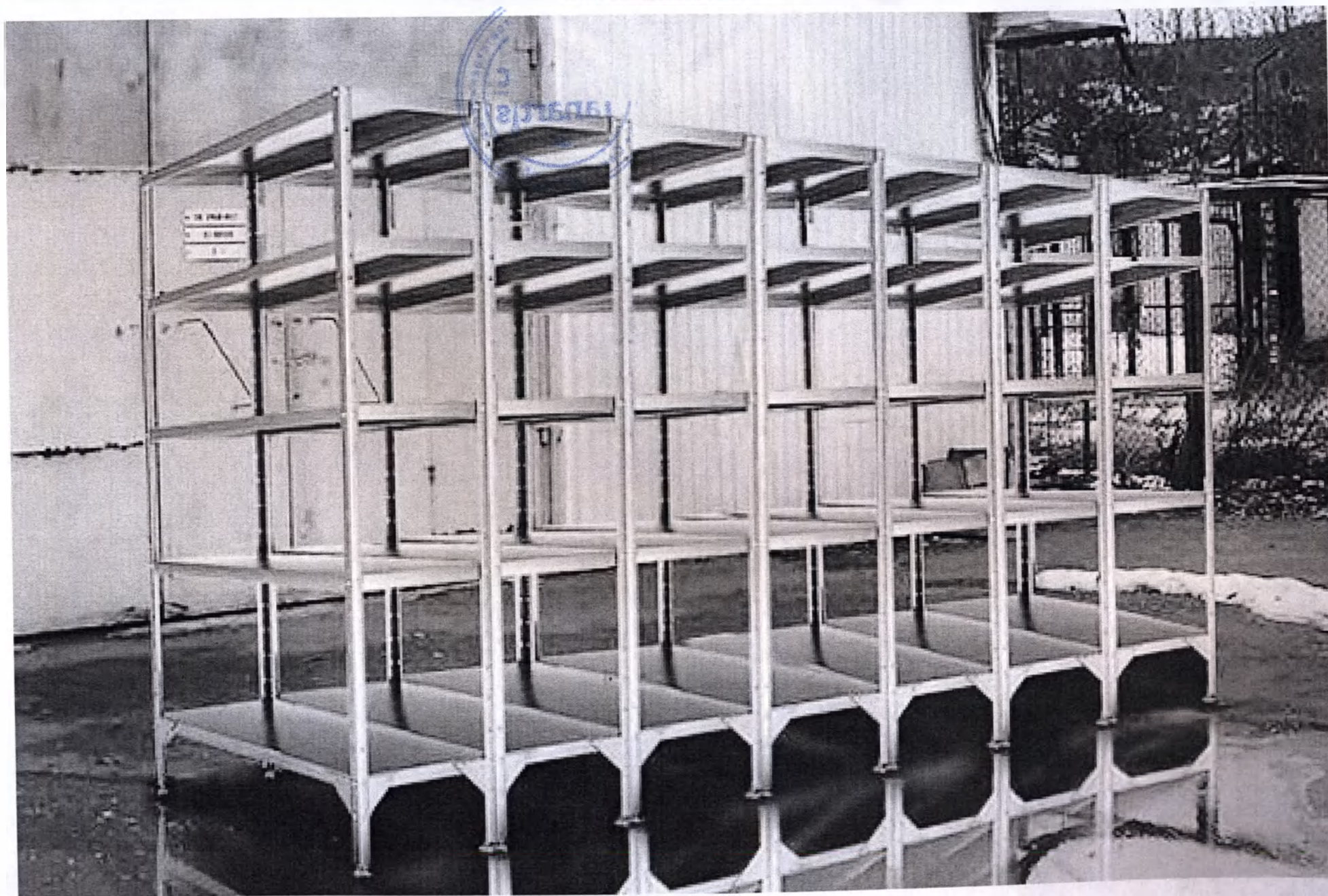
15. Стационарные стеллажи для хранения трупов Tanartis на 35 мест для скользящих поддонов и поддонов на колесах
