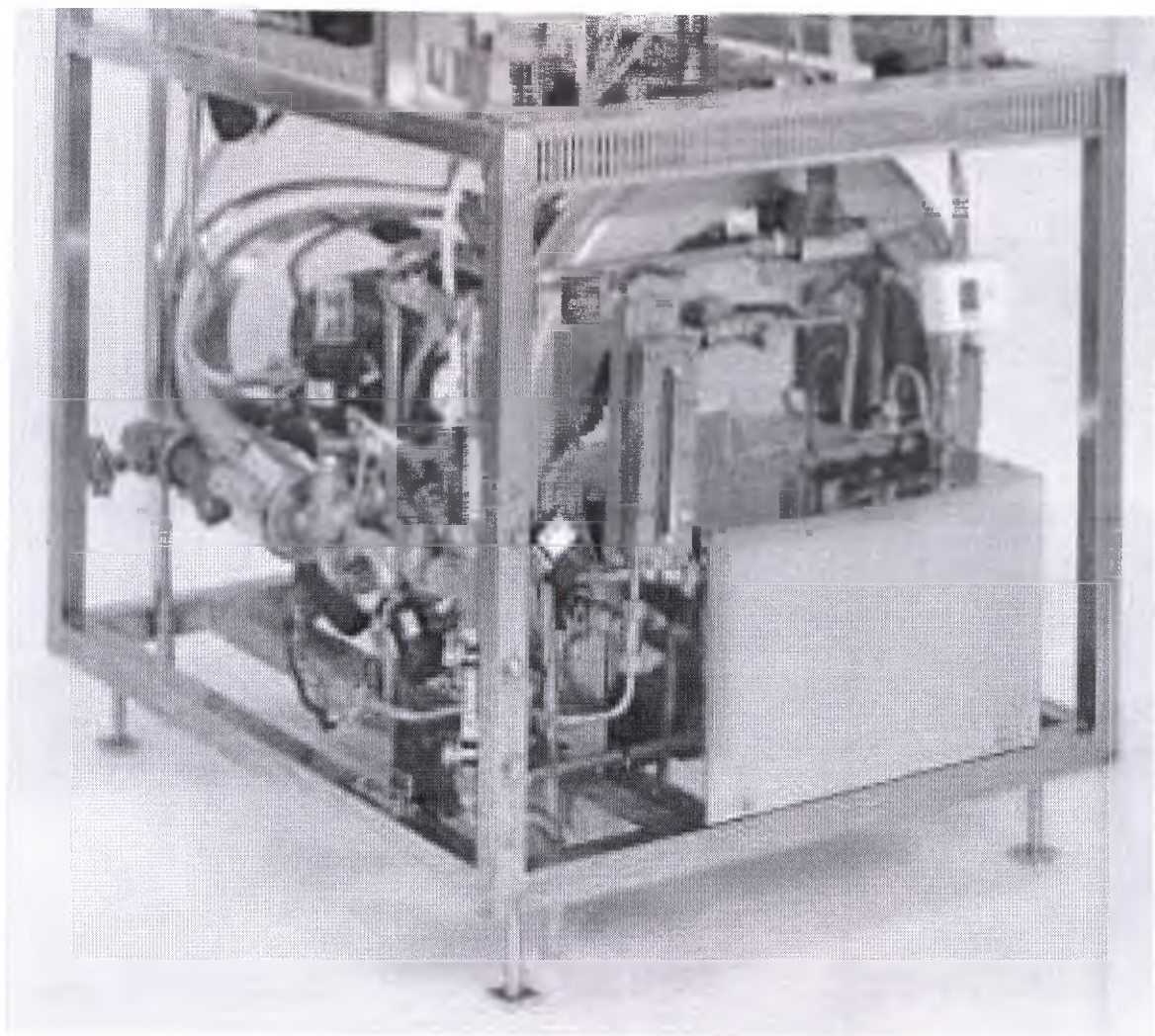
Фото 11. Парогенератор серии ED
