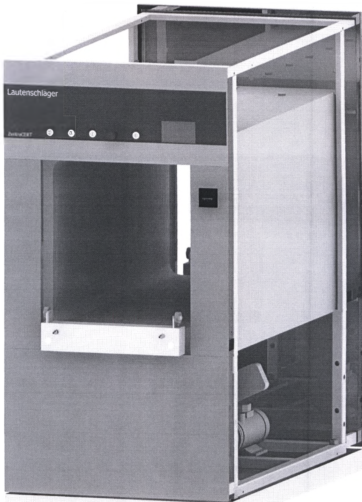
Фото 6. Стерилизатор паровой Zentracert, вариант исполнения 6200
