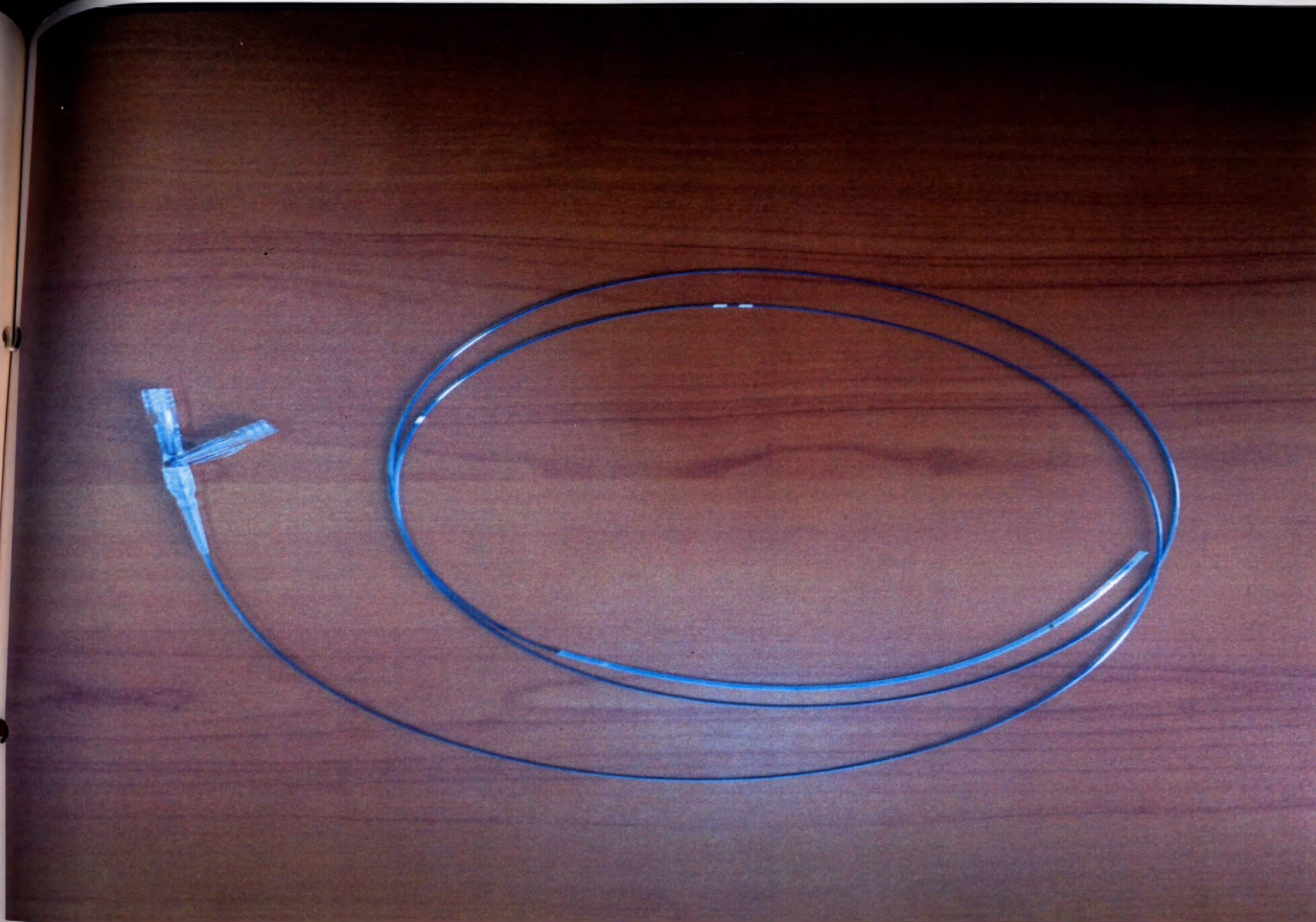
Катетер баллонный дилатационный Sterling Over-The-Wire, диаметр баллона от 1,5 мм до 10 мм, длина катетера 40 см, 80 см, 90 см, 135 см, 150 см (общий вид)
