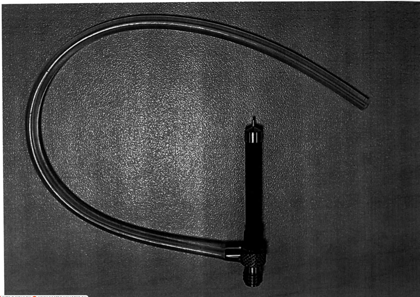
Фото 5 - Зонд закрытый контактный CP 1 мм (Closed contact probe - CP 1 mm)
