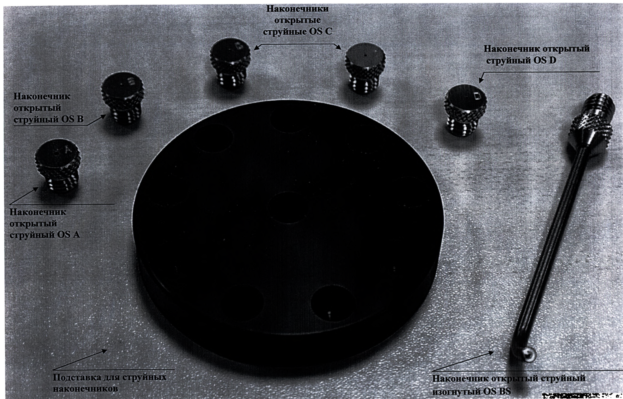
Фото 3 - Набор наконечников открытых струйных
