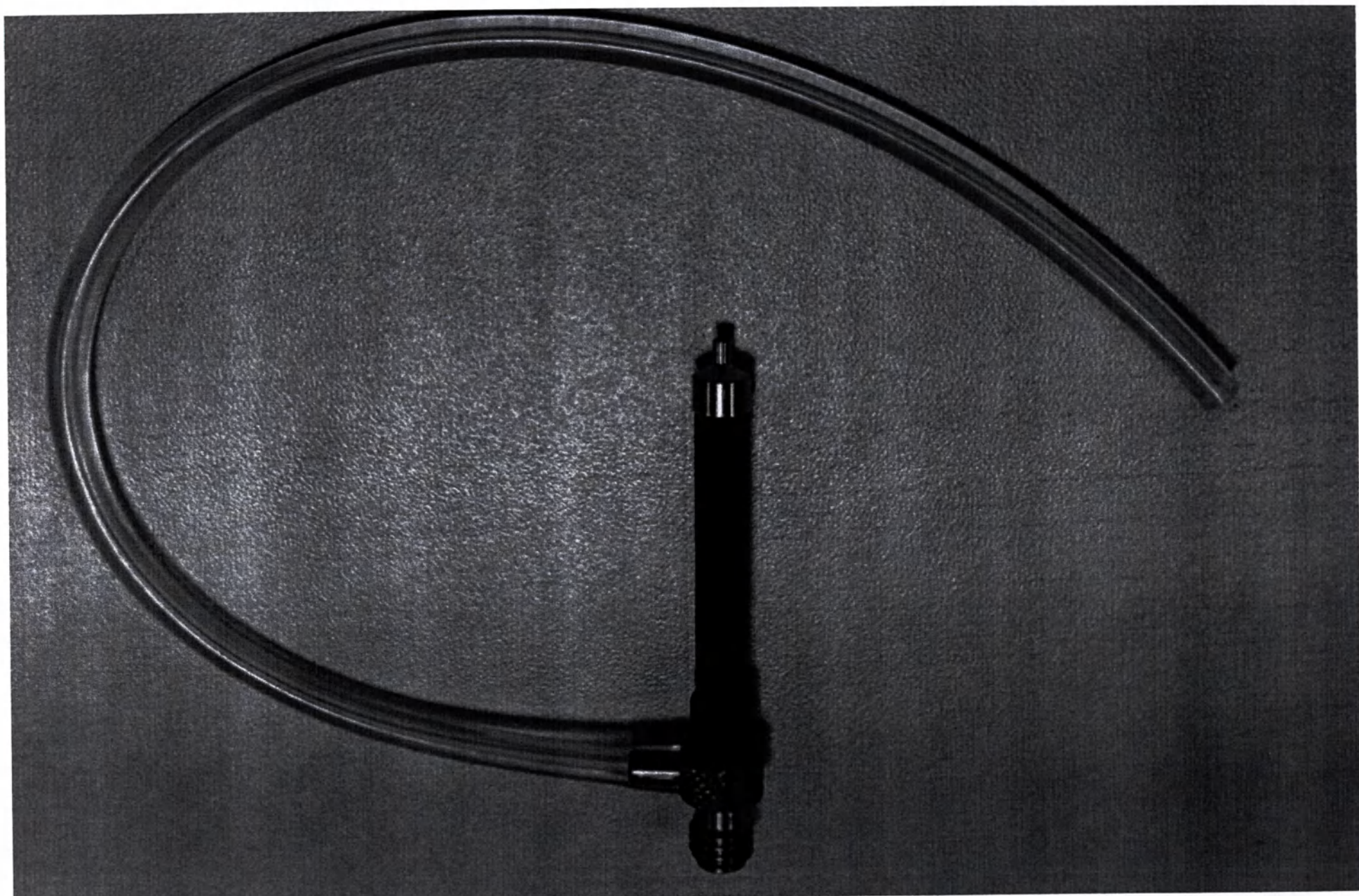
Фото 6 - Зонд закрытый контактный CP 2 мм (Closed contact probe - CP 2 mm)
