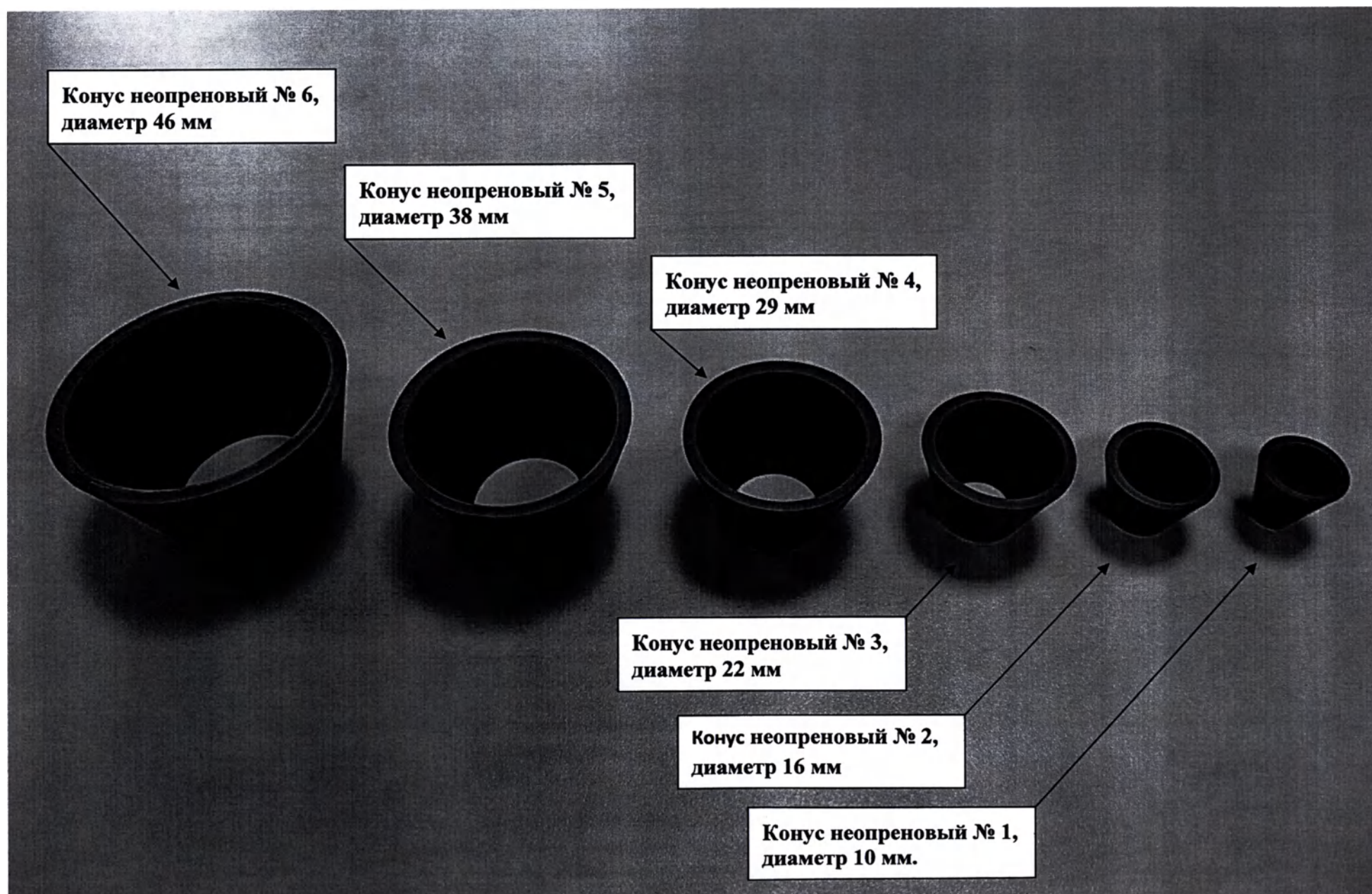
Фото 31 - Комплект конусов неопрезовых из 6 штук (Neoprene cones, a set of 6)
