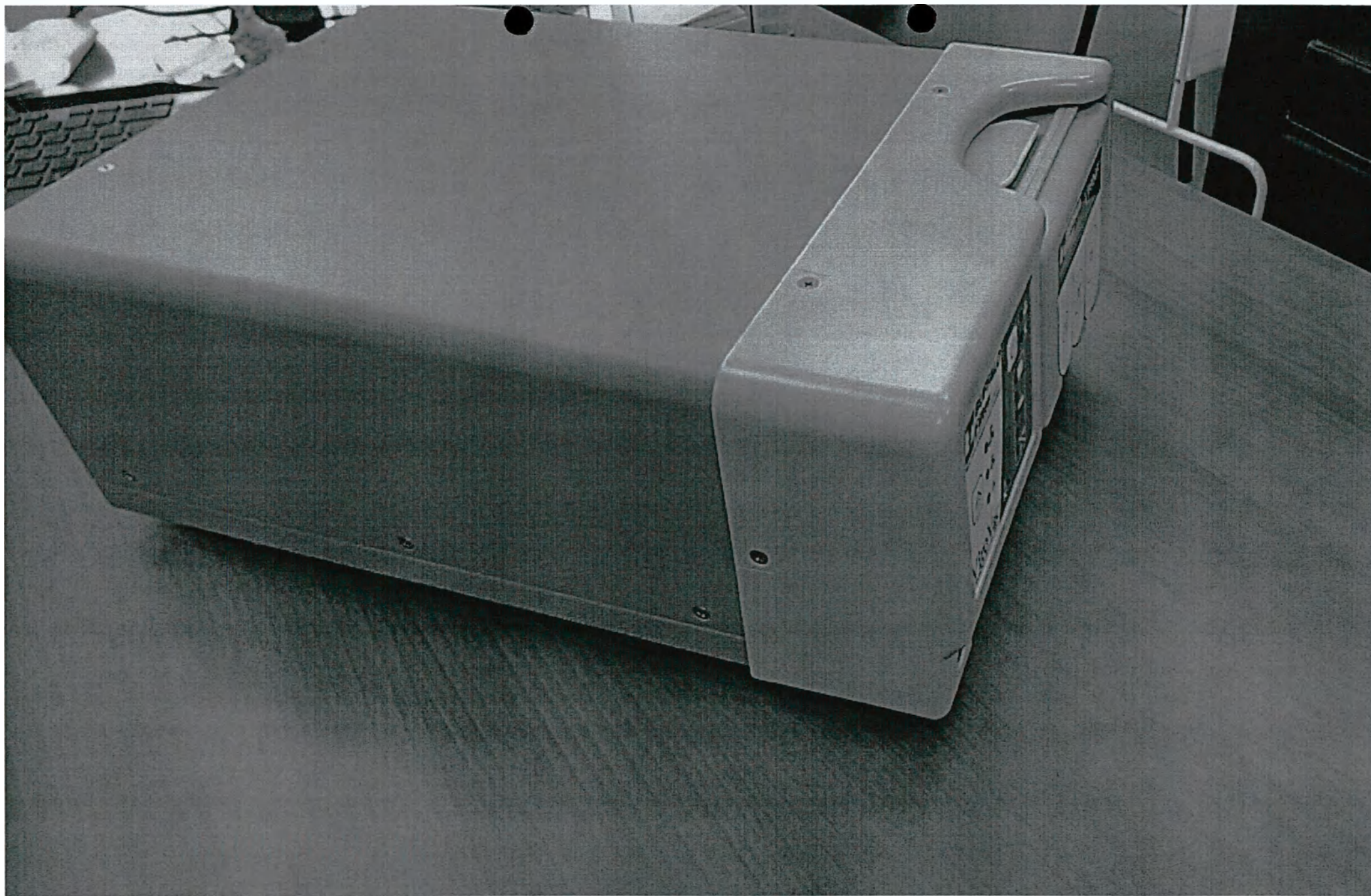
20. Дымоотсос, ширина 25,0 см, глубина 30,0 см, высота 22,0 см.
