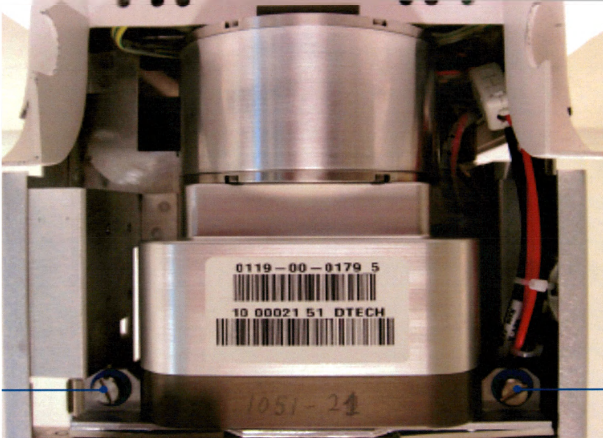
Компрессор DUAL HEAD Scroll Assembly 750 RPM
