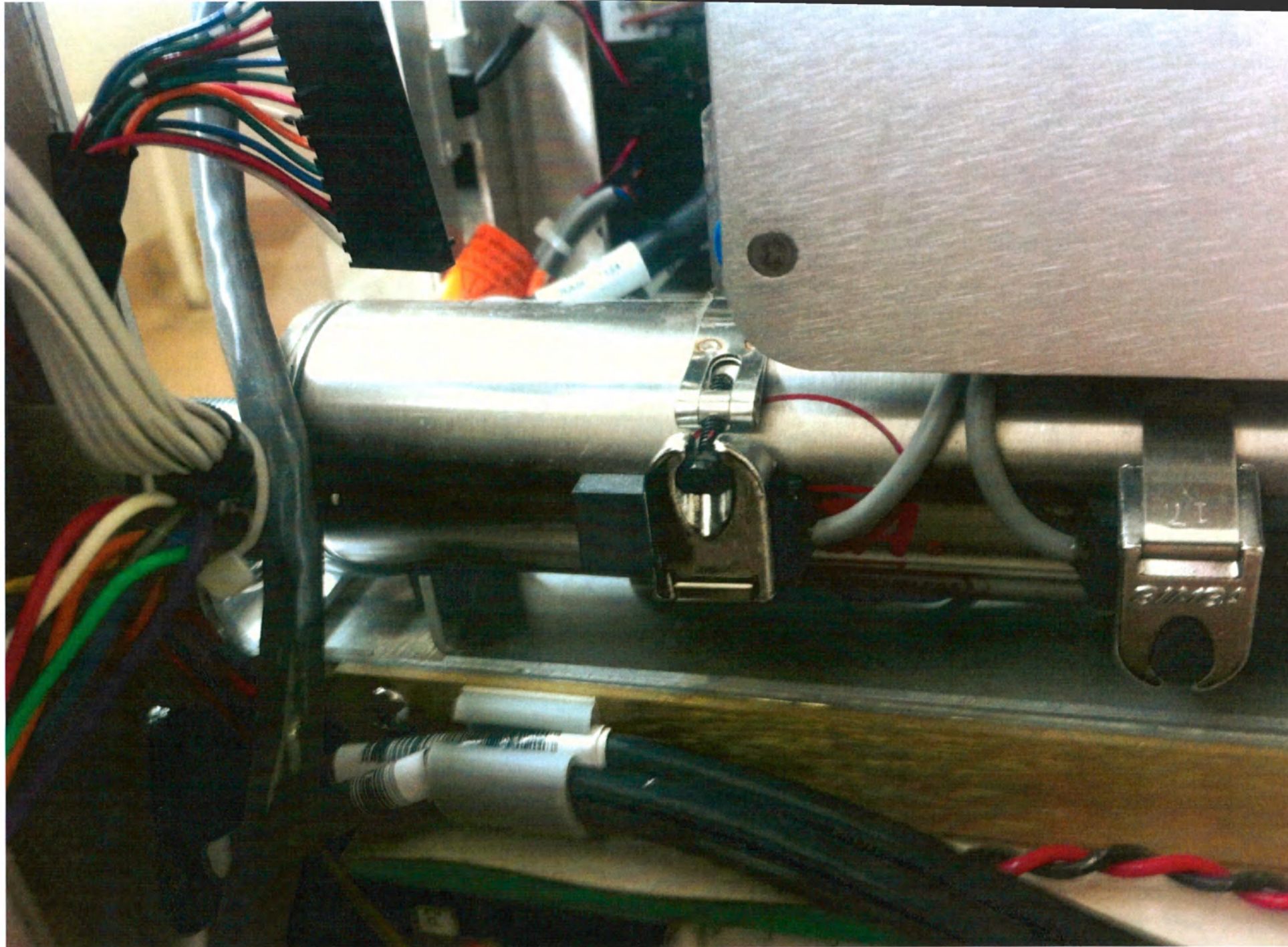
Цилиндр подачи гелия пневматический BIMBA cylinder
