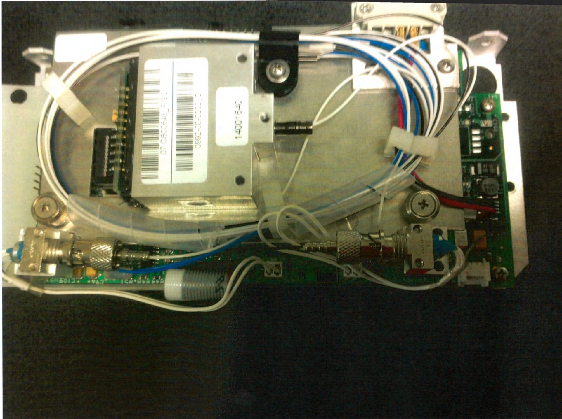
Фиброоптические компоненты (лампочки L1-B) + Фиброоптические компоненты (лампочки L1-w)
