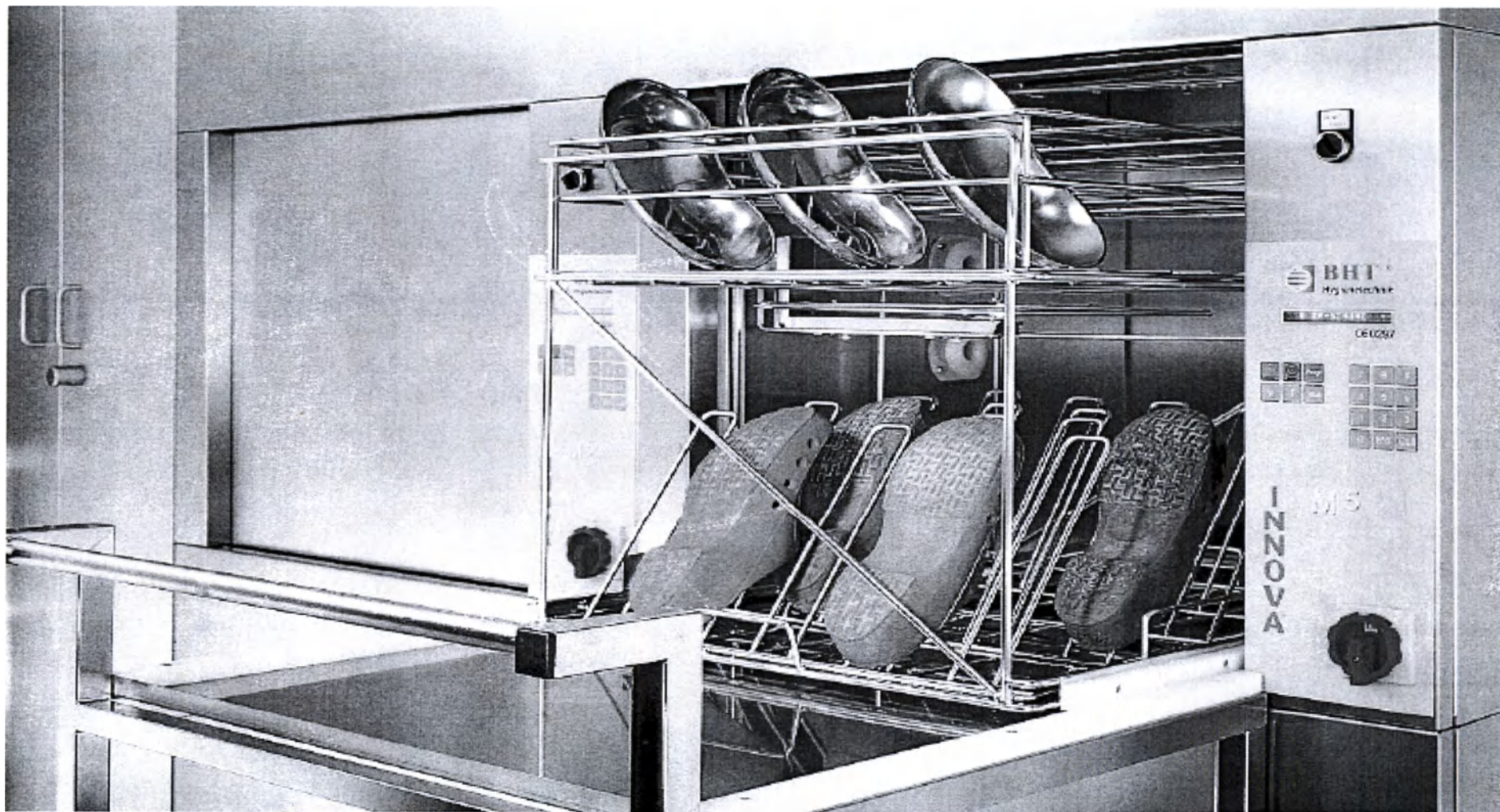
МАШИНА МОЮЩЕ-ДЕЗИНФИЦИРУЮЩАЯ INNOVA M5 - 1
