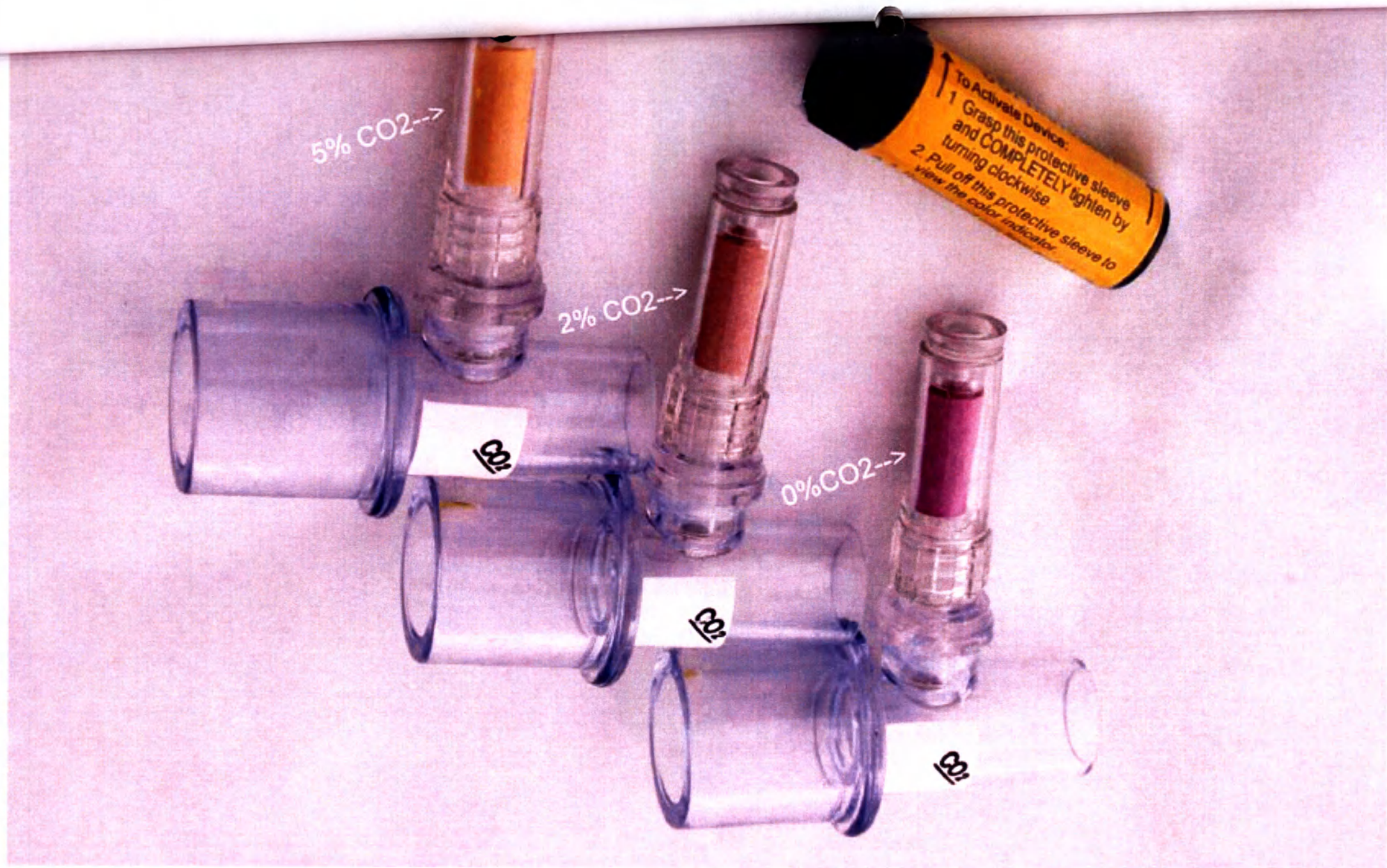
SC-200 – StatCheck II CO2 Детектор
