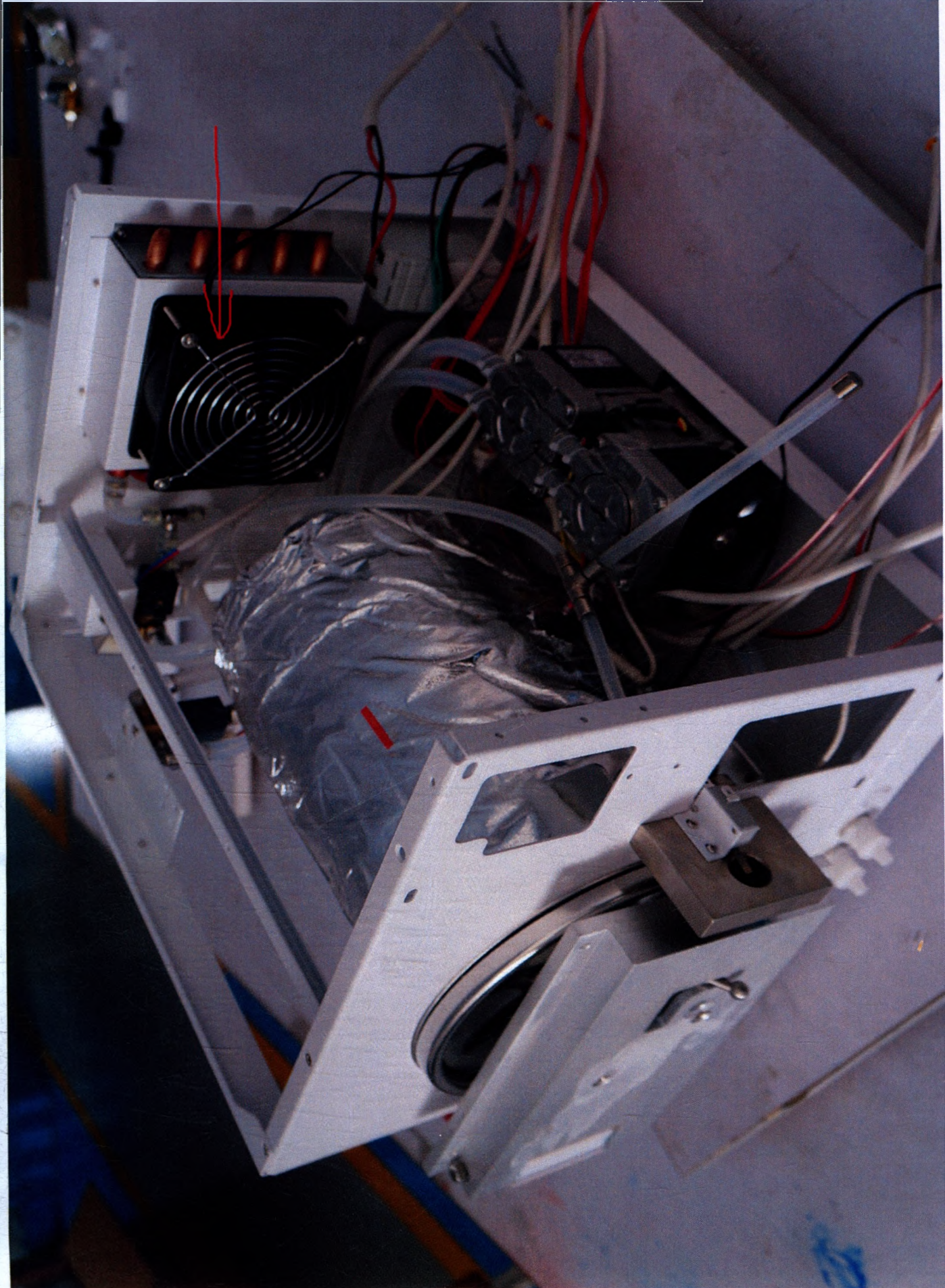
Охлаждающий модуль
