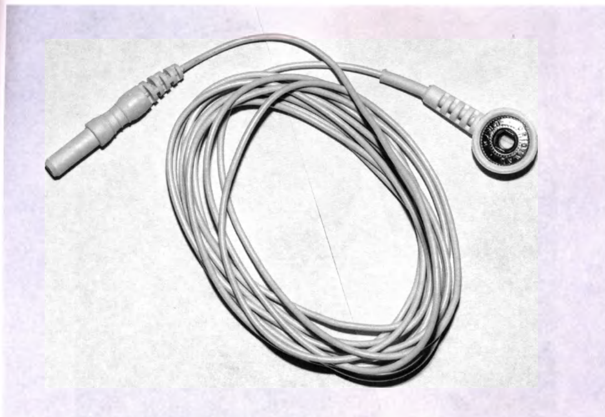
Кабель для подключения одноразовых электродов с коннектором «кнопка», touch-proof (2 м) – белый
