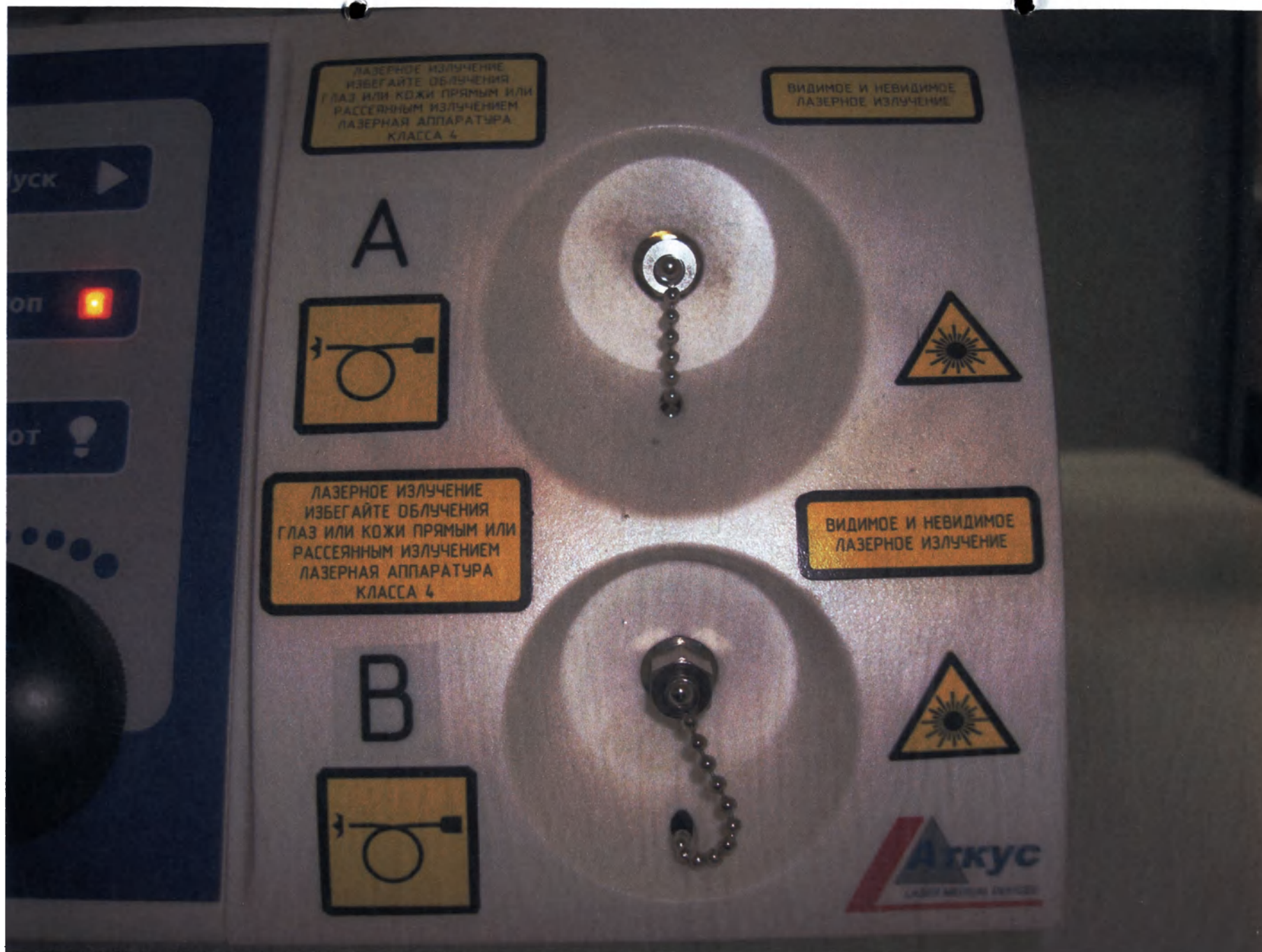
Аппарат лазерный медицинский Латыс-М вид спереди
