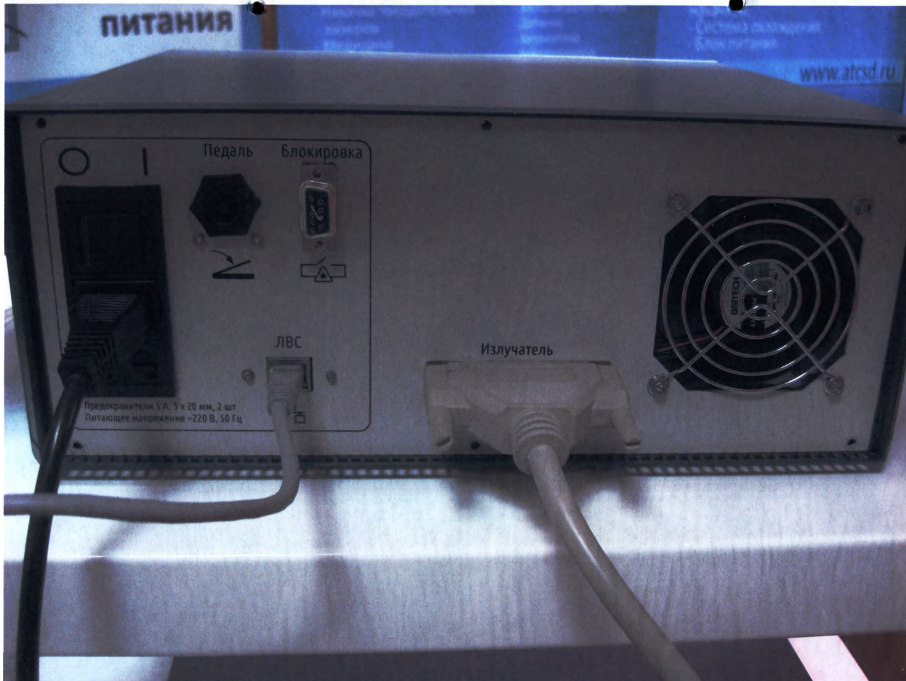
Блок питания аппарата светодиодного медицинского Латус-М вид сзади
