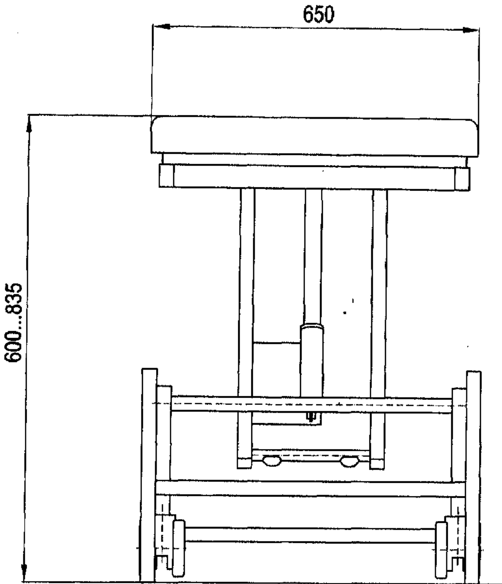
Рис. 1. – Схема-чертеж. модель СМ- «Техстрой 1» односекционный, ЭЛЕКТРОННАЯ КОПИЯ ОФОРМЛЕНА ЦЕНТРОМ ИСПЫТАНИЙ И РЕГИСТРАЦИИ МЕДИЦИНСКИХ ИЗДЕЛИЙ вид спереди.
