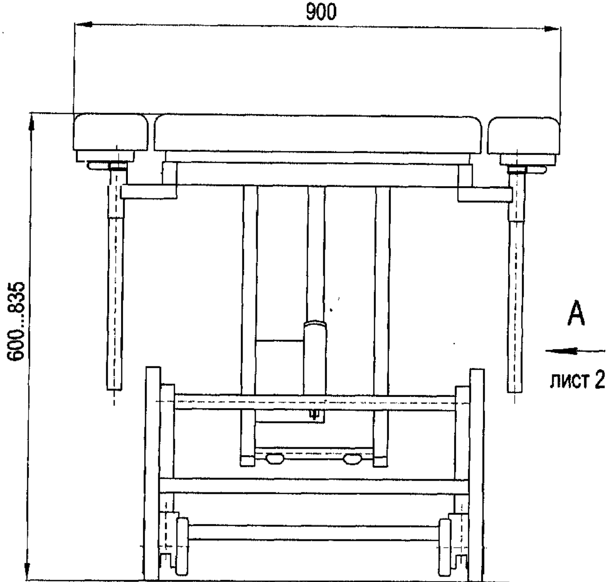
Рис. 5. – Схема-чертеж, модель СМ- «Техстрой 3» трехсекционный,
