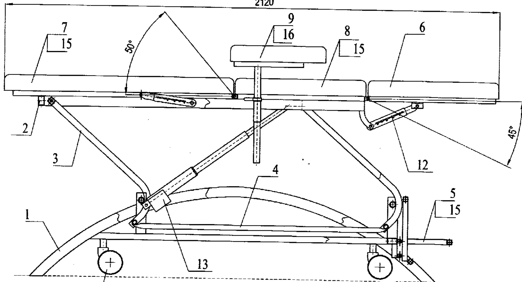
Рис. 6. – Вид сбоку.
