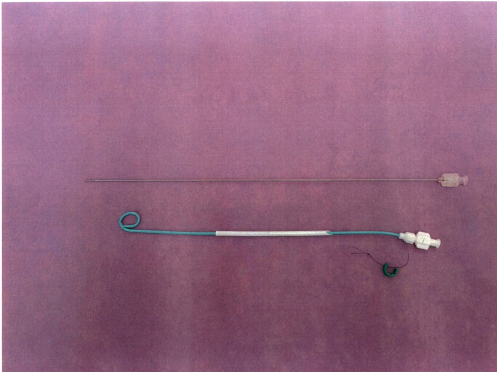
Рис.5.1.Катетеры дренажные одноразовые стерильные с наконечником в виде замкнутой петли и фиксирующей нитью (по Селдингеру) в наборах:
