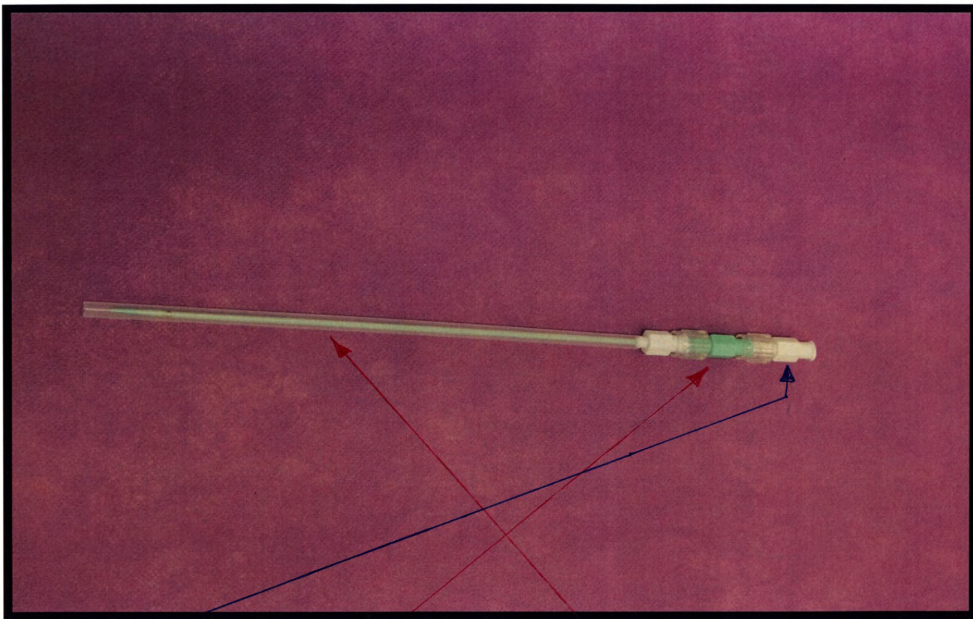
Рис. 10.3. Канюля жесткая металлическая, расширитель, ножны с гидрофильным покрытием (с рентгеноконтрастной меткой) в наборе для установки дренажного катетера одноразового стерильного: HD-N6410.
