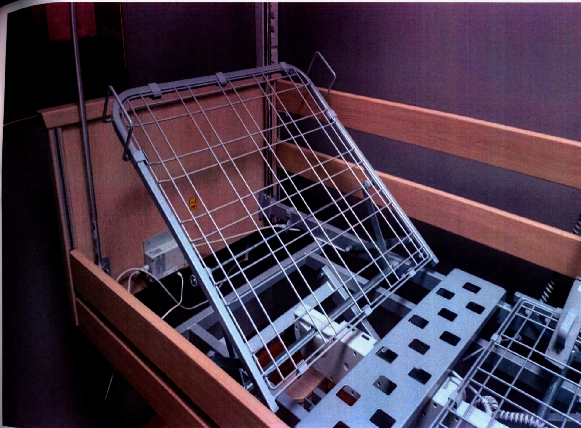
Спинная секция. (Movita casa и Movita )
