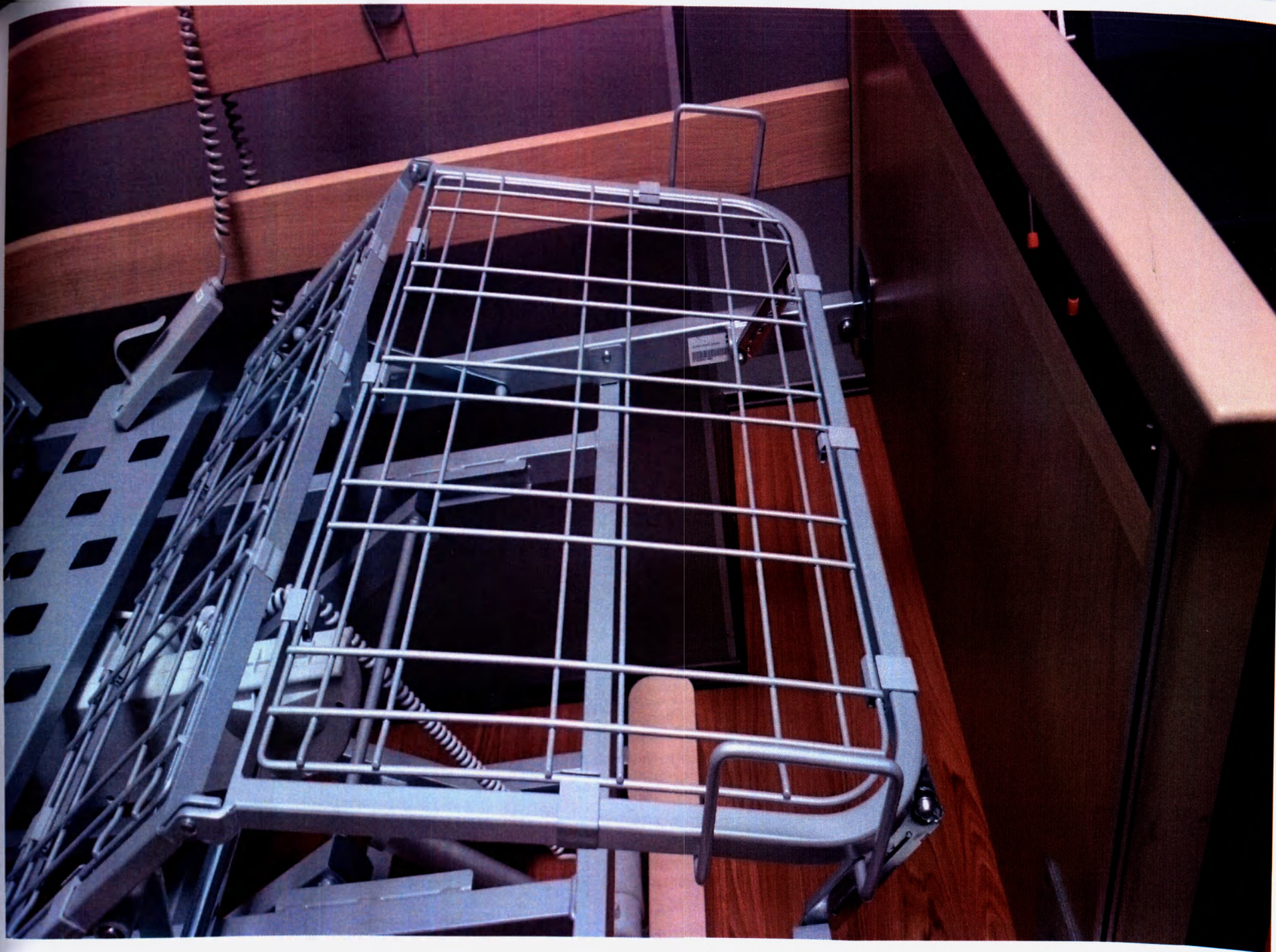
Ножная секция. (Movita casa и Movita )
