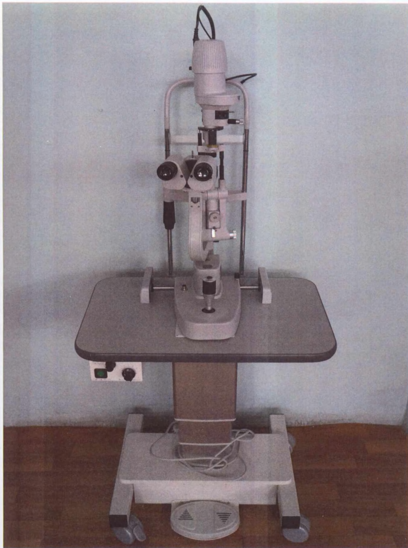
Щелевая лампа ЛС-04-01 «Зенит»
